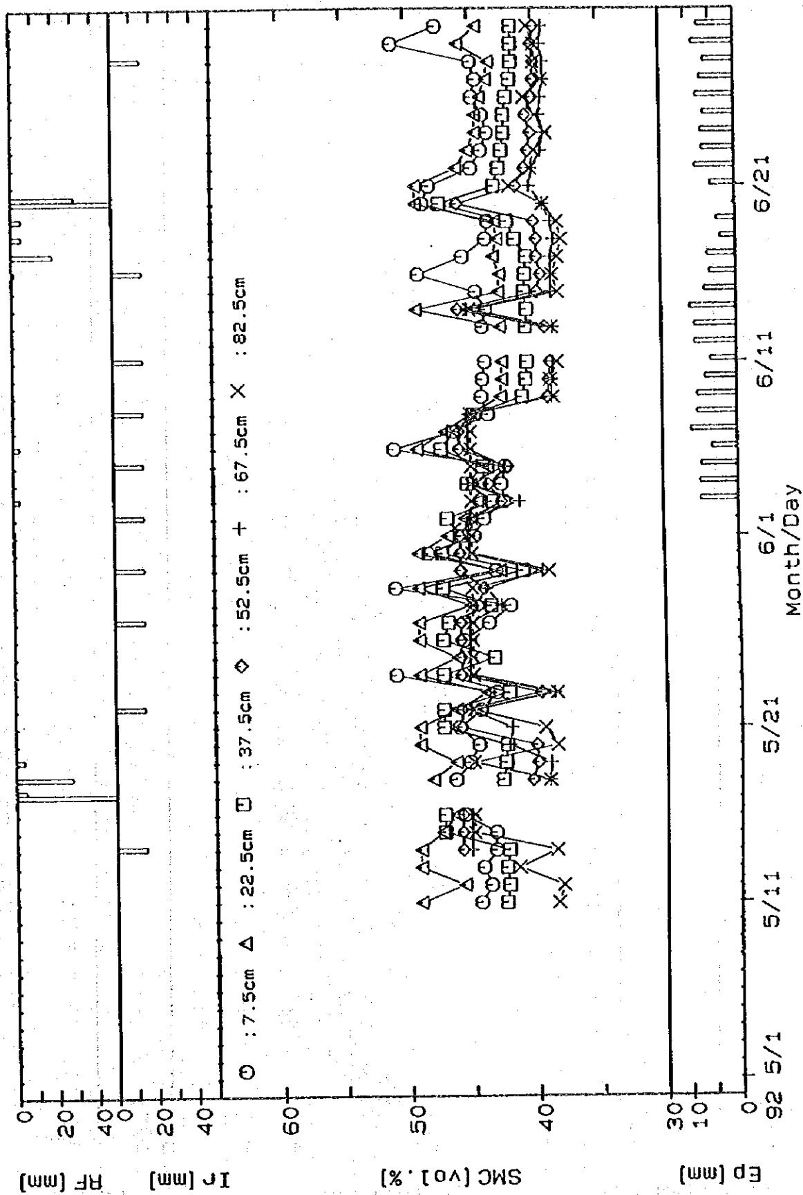
図36 土壌水分量の経時変化 (トマト圃場 15. No. 1)
