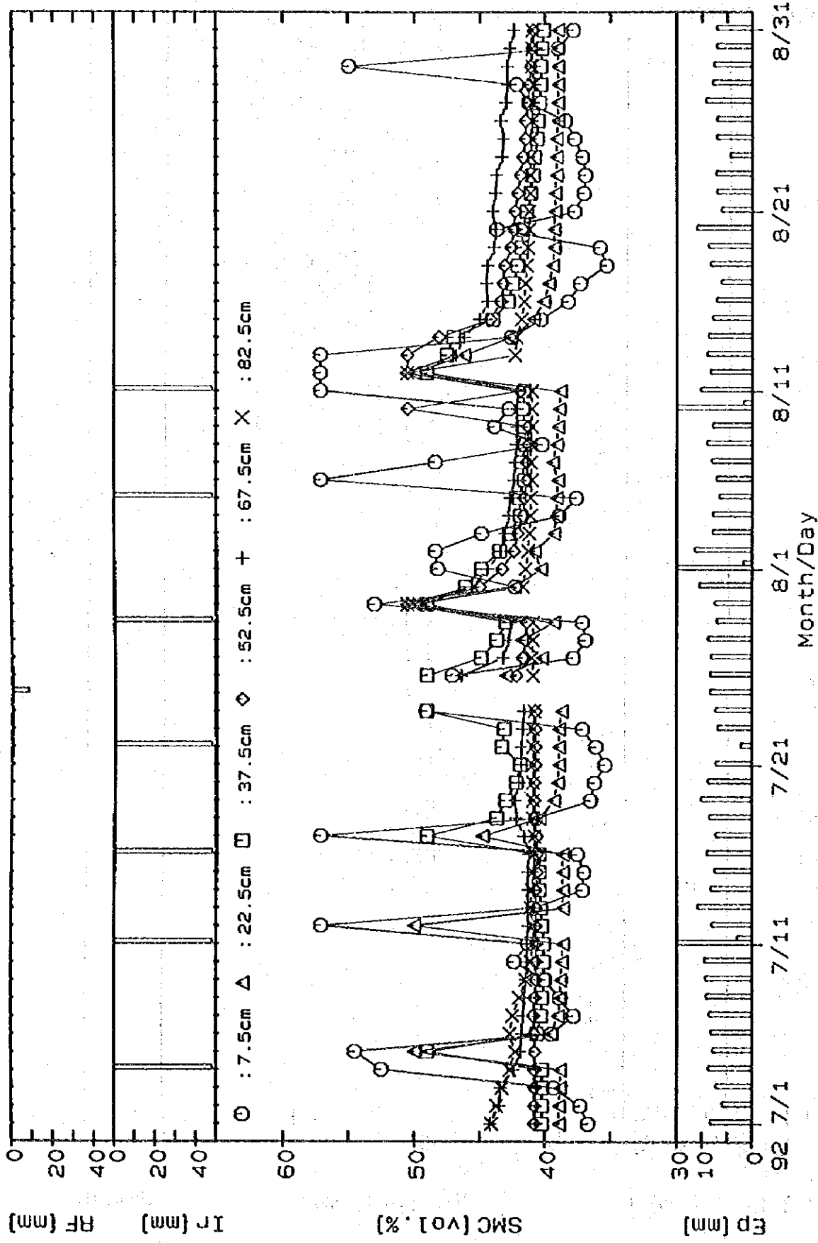
図51 土壤水分量の経時変化 (ダイズ圃場 30. No. 2)
