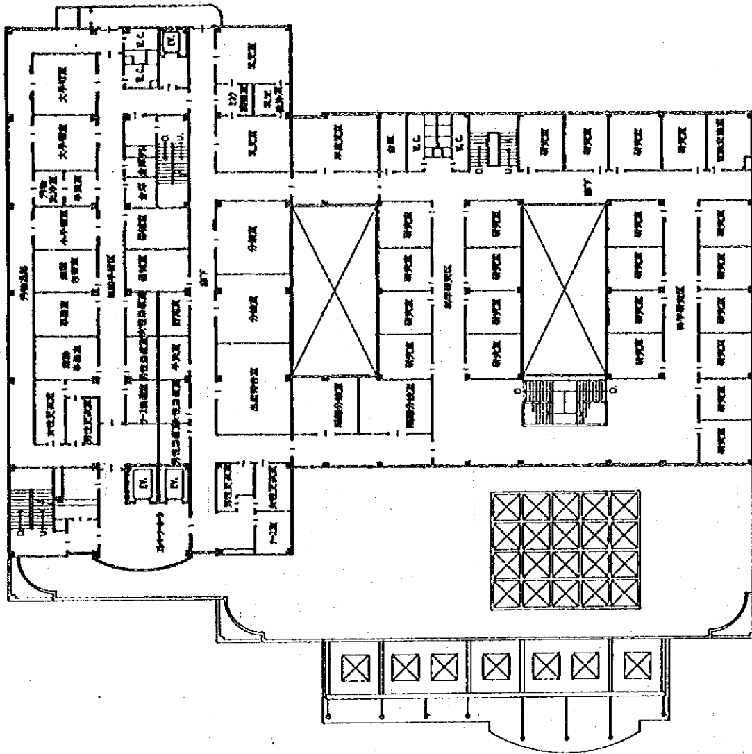
国会议事堂議院センター 3階平面図 外装、新機、改修 24:30
