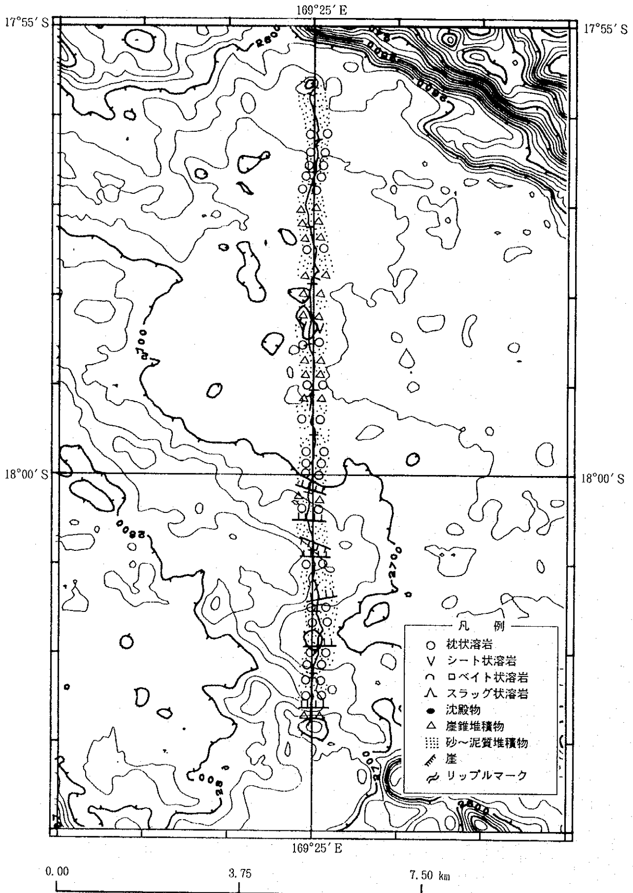
添付 第 4 図 FDCルートマップ (94SFDC08測線) (5) (ヴェイトトラフ中央部)
