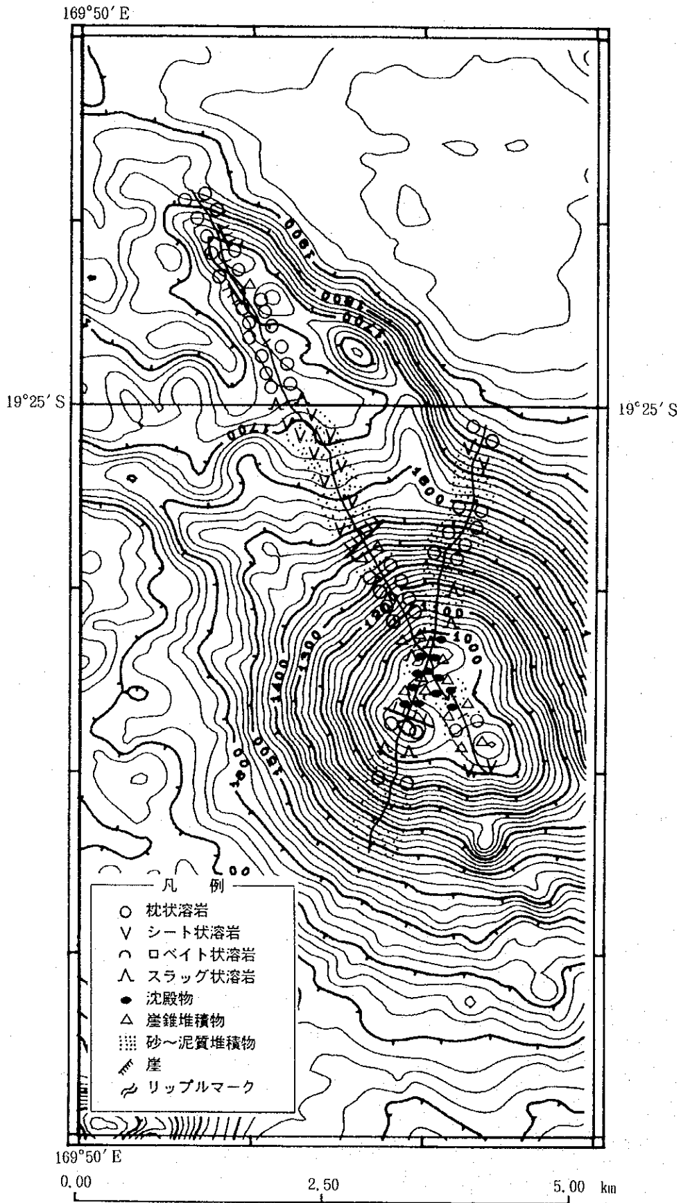
添付 第 4 図 FDCルートマップ (94SFDC04, 05測線) (3) (94S02海山)
