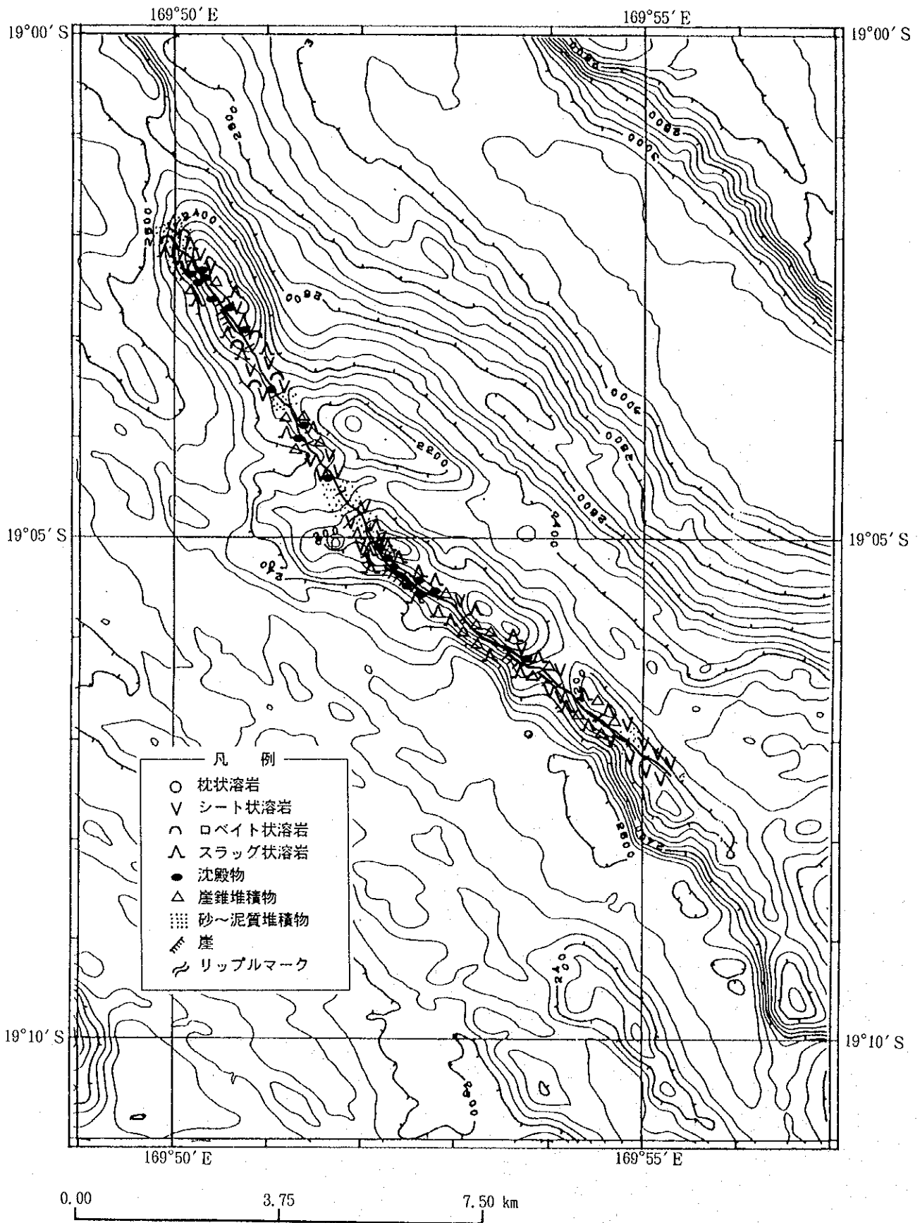
添付 第 4 図 FDCルートマップ (94SFDC01測線) (1) (エロマンガベズン中央部)
