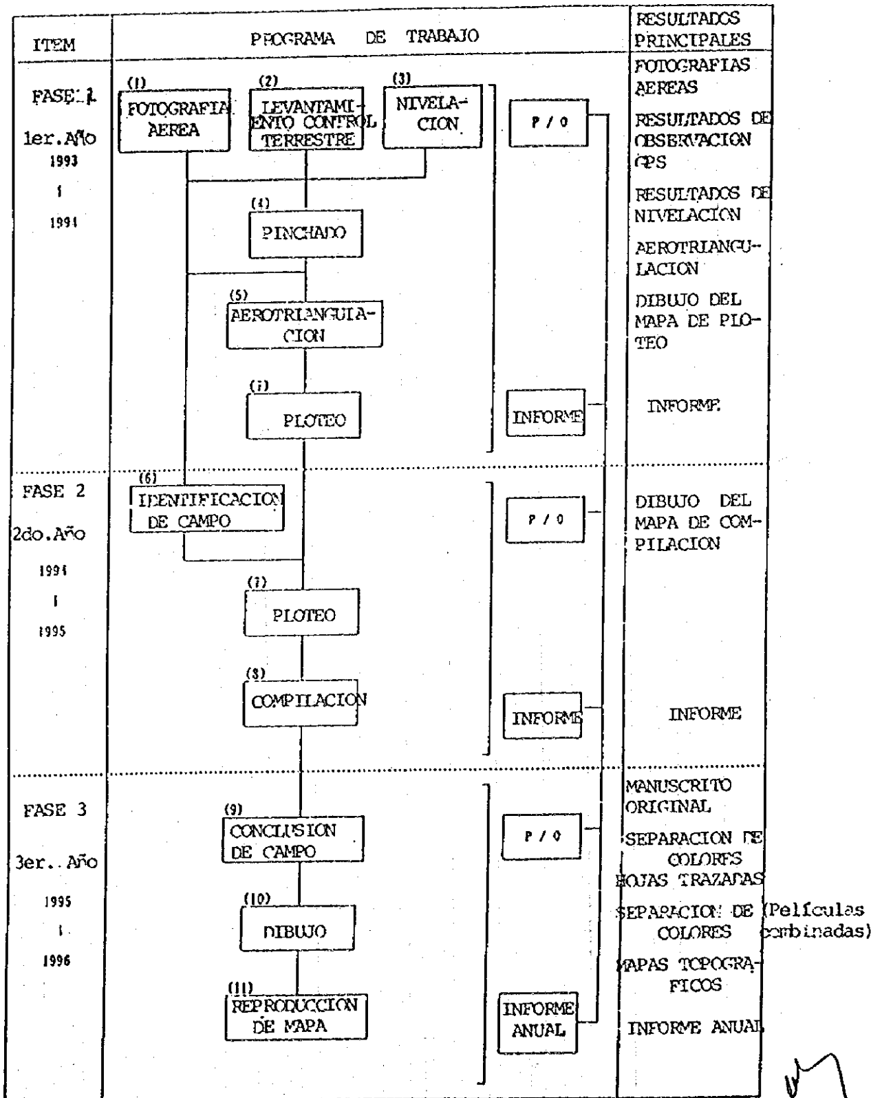
FIGURA 5 DIAGRAMA PARA LA PRODUCCION DE MAPAS TOPOGRAFICOS
