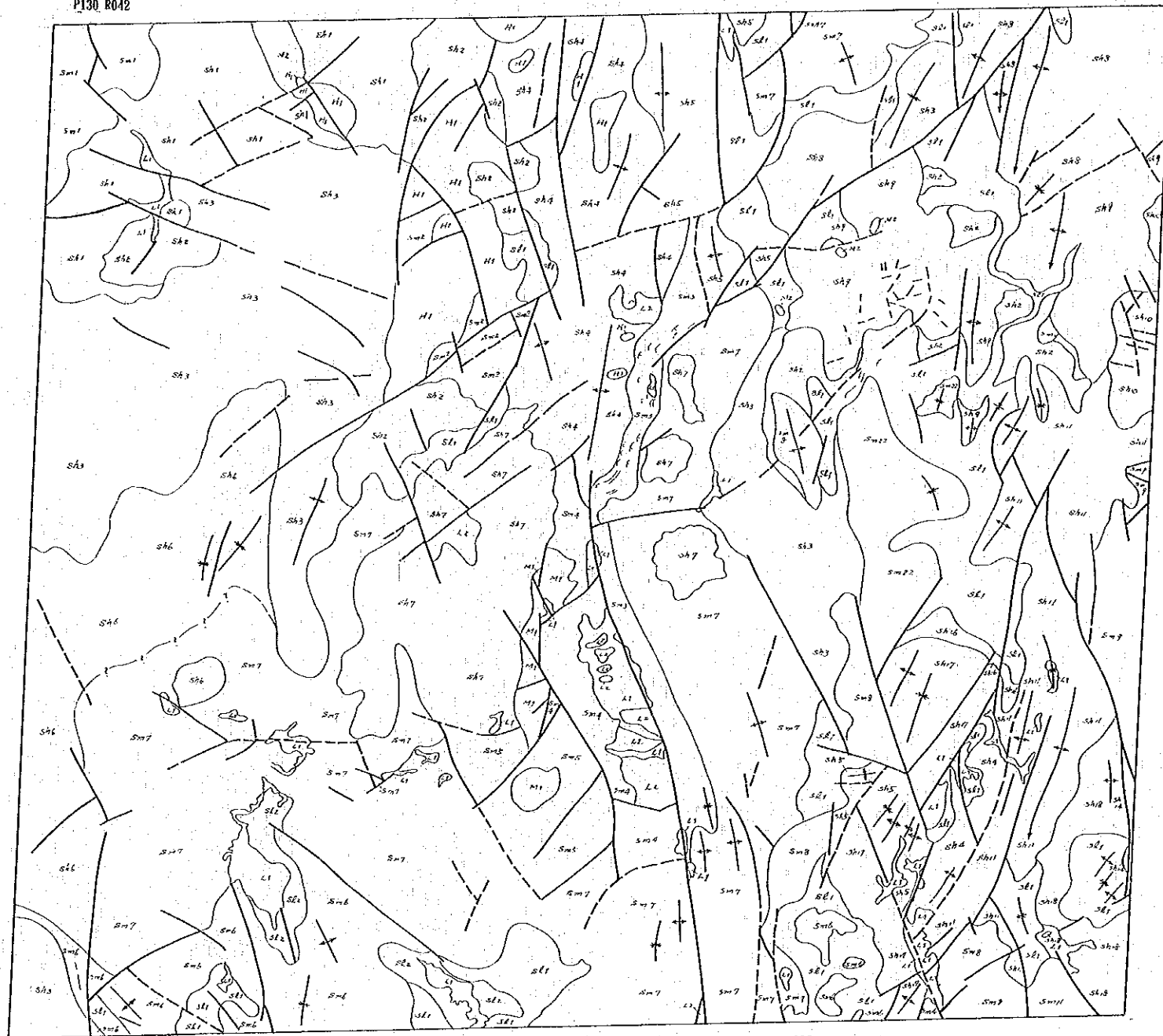
付图2-13 卫星画像判读结果图(云南省禄武地区 P130, R042) 缩尺 1:500,000
