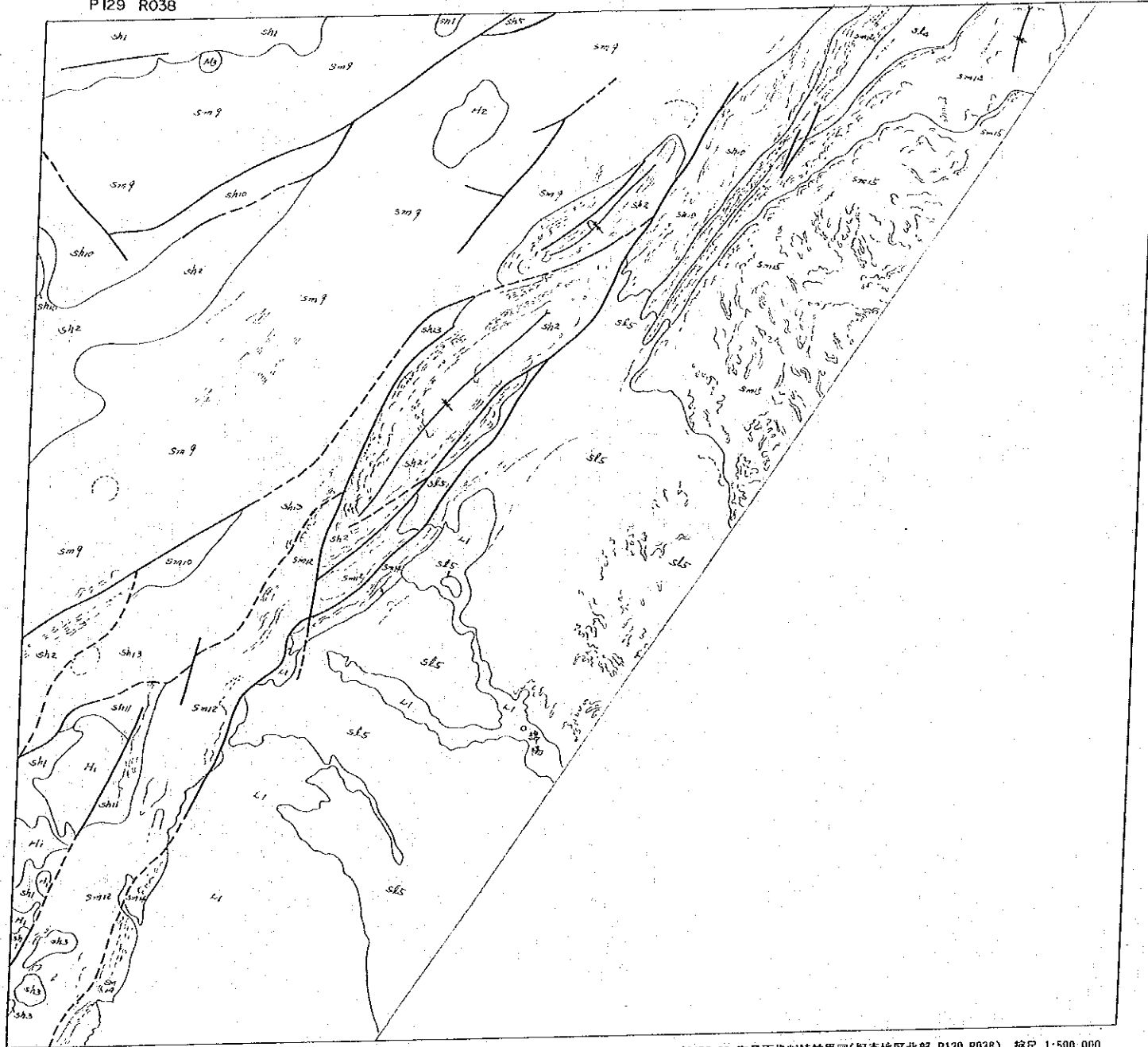
村图2-26 卫星图像判读结果图(调查地区北部 P129, R038) 缩尺 1:500,000.
