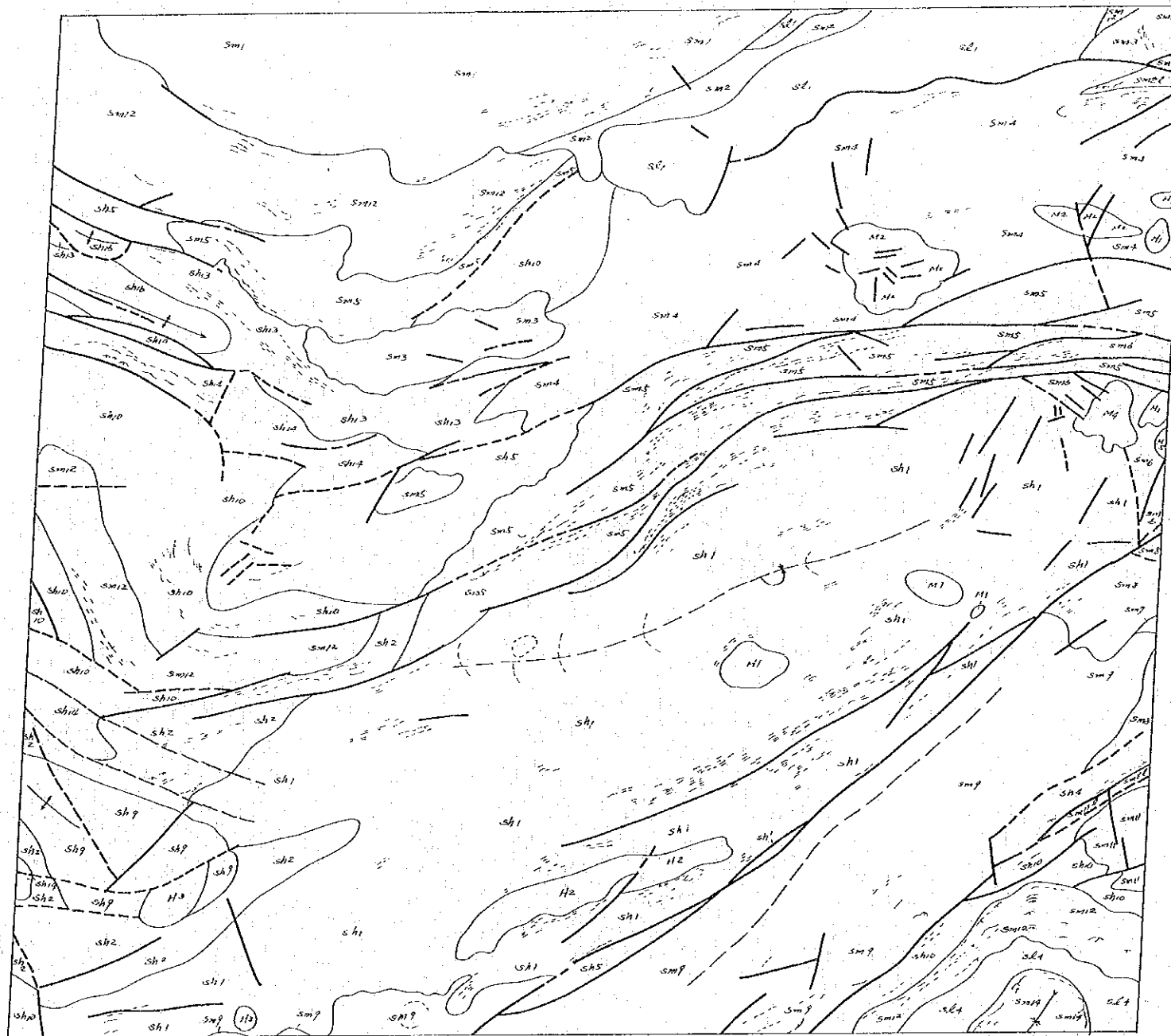
付圖2-22 衛星遙像判讀結果圖(樞查地區北部 P129, R037) 縮尺 1:500,000
