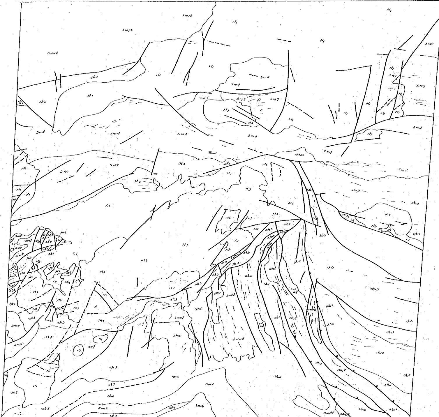
付图2-21 卫星图像判读结果图(调查地区北部 PI37, R037) 缩尺 1:500,000
