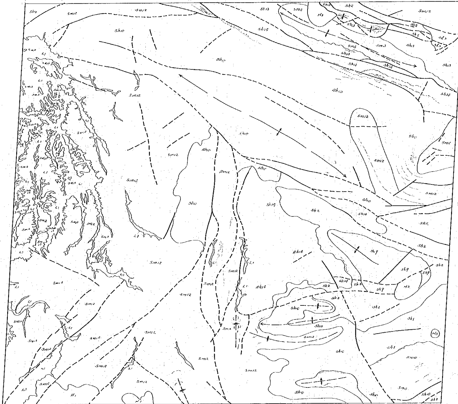
付圖2-23 衛星影像判讀結果圖(棋盤地區北部 P130, R037) 縮尺 1:500,000
