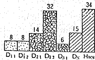
台風経路頻度図
