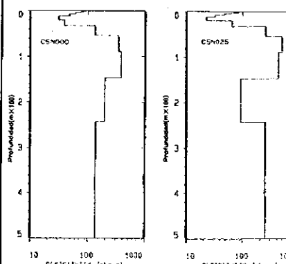
RESULTADOS DE LA INVERSION PARA EL MODELO MULTISTRATIFICADO
