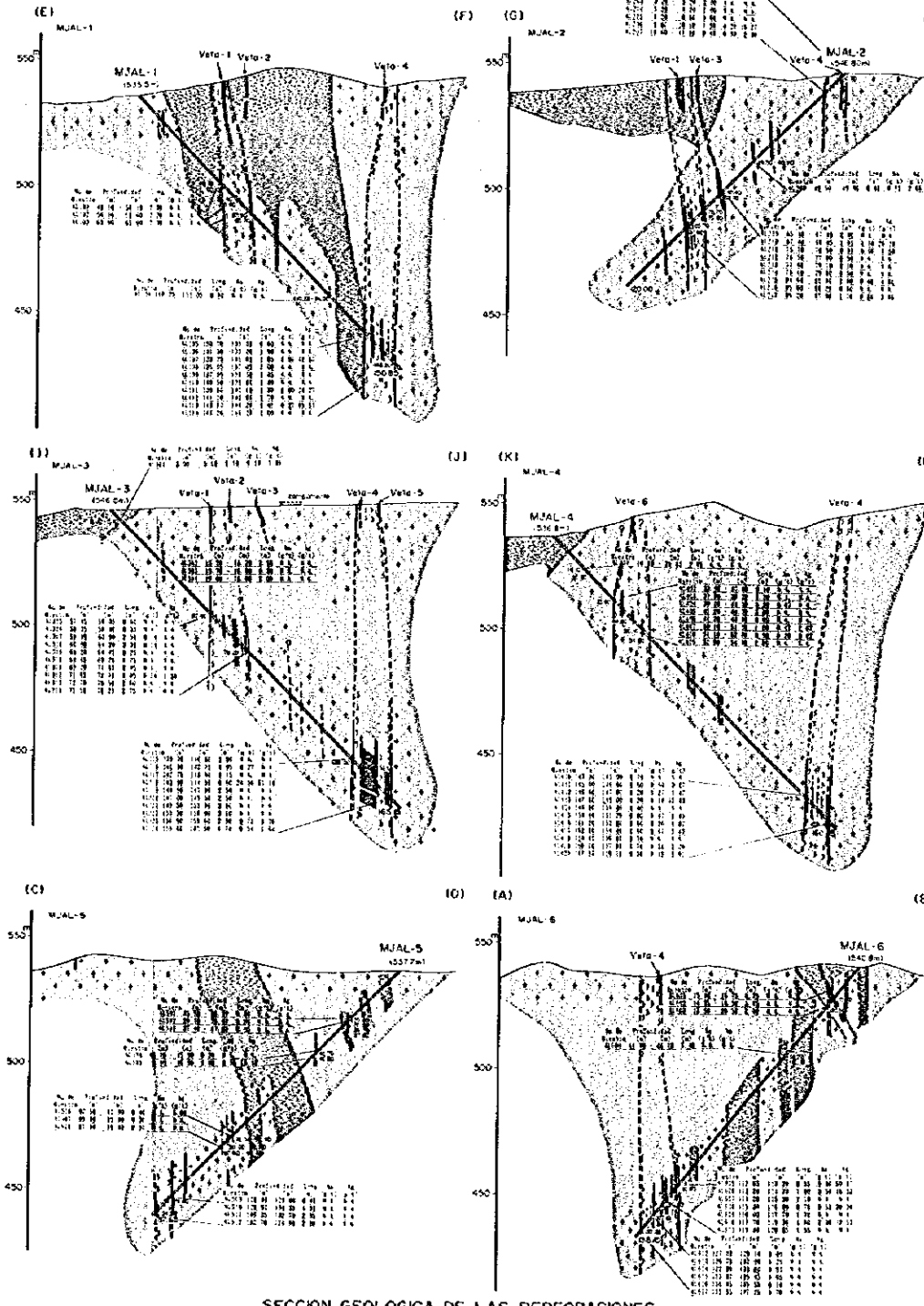
SECCION GEOLOGICA DE LAS PERFORACIONES
