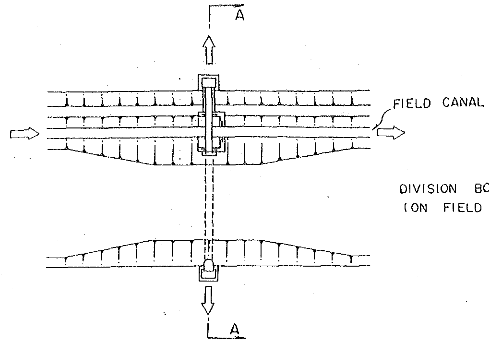
PLAN SCALE-A
