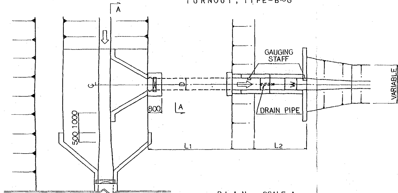
PLAN SCALE-A
