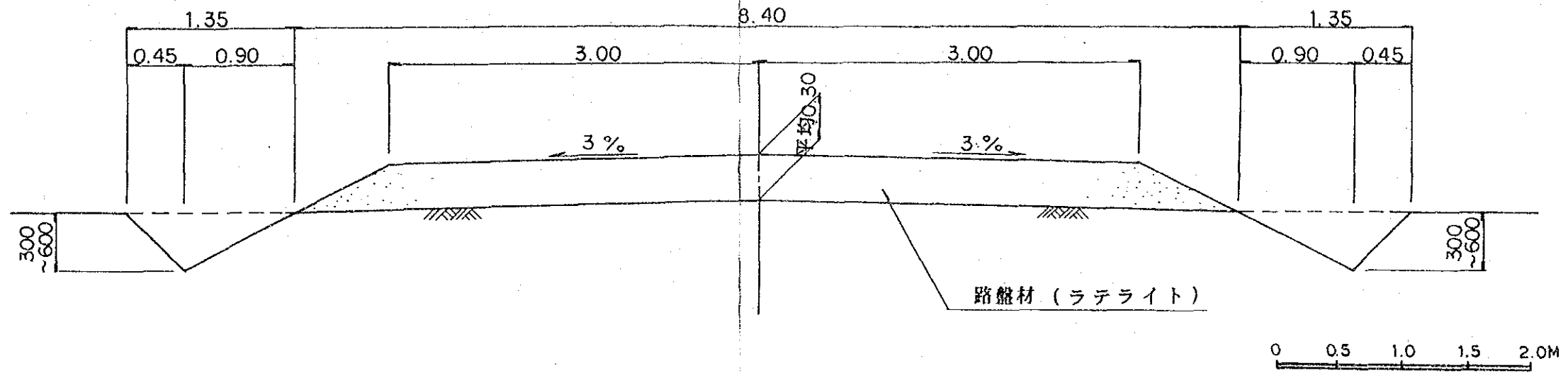
横断管埋設標準図 縮尺 1:20
