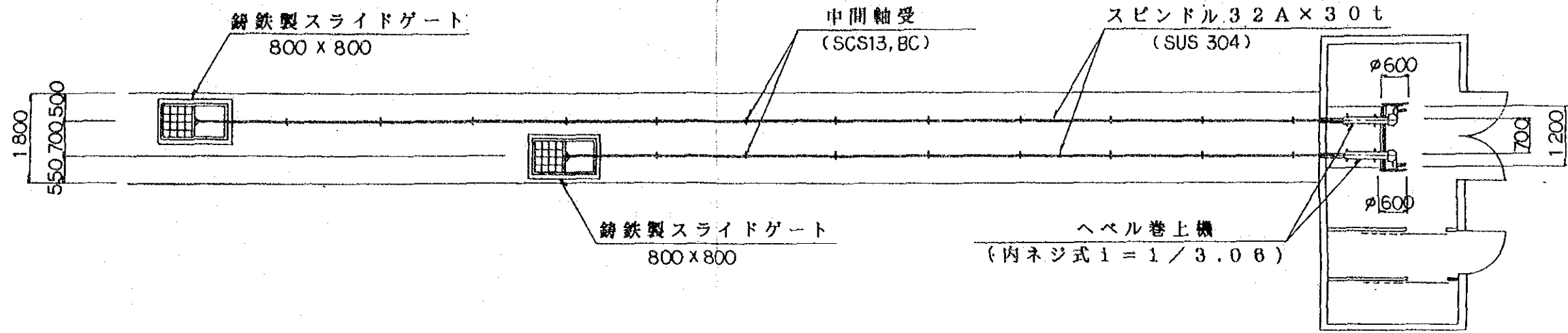
平面図 縮尺 1:100
