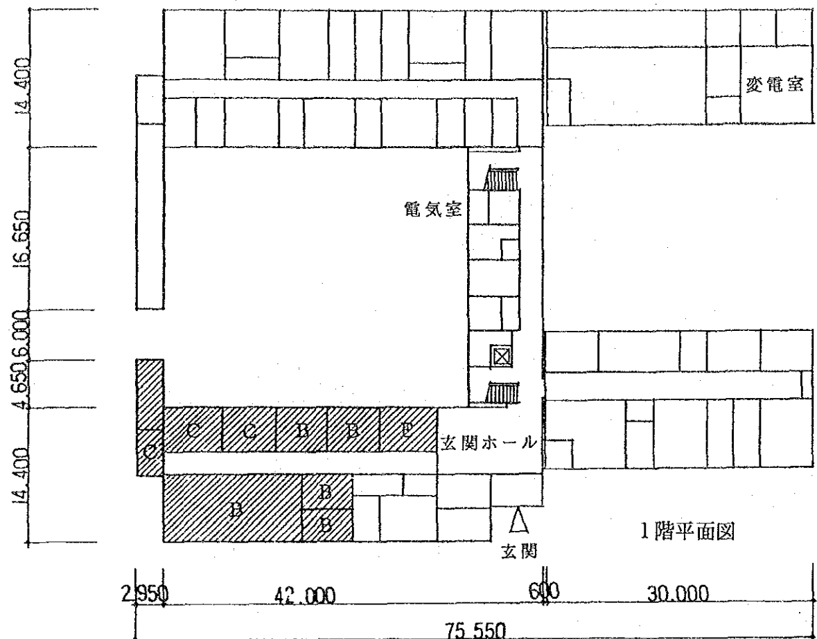
図 3.5 実験室配置図 (求是楼平面図)
