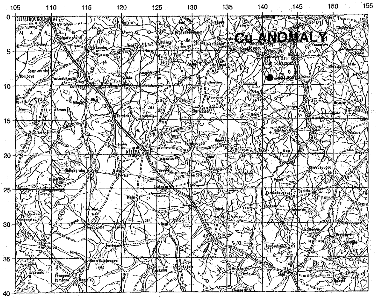
図 67 ケレヤ地区地化学探査解析結果図 (Cu)
