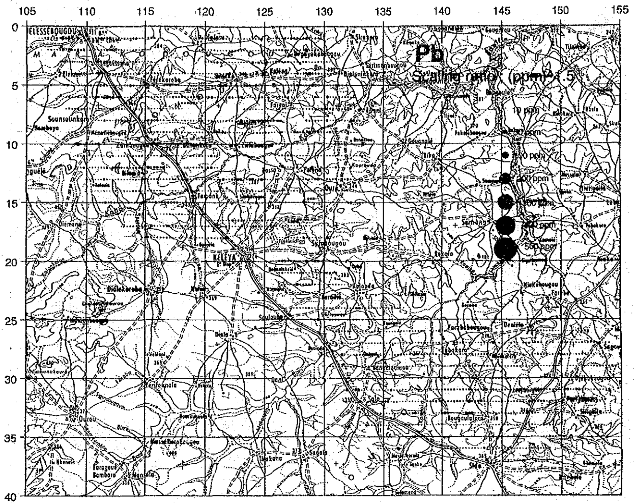
図 68 ケレヤ地区地化学探査結果図 (Pb)
