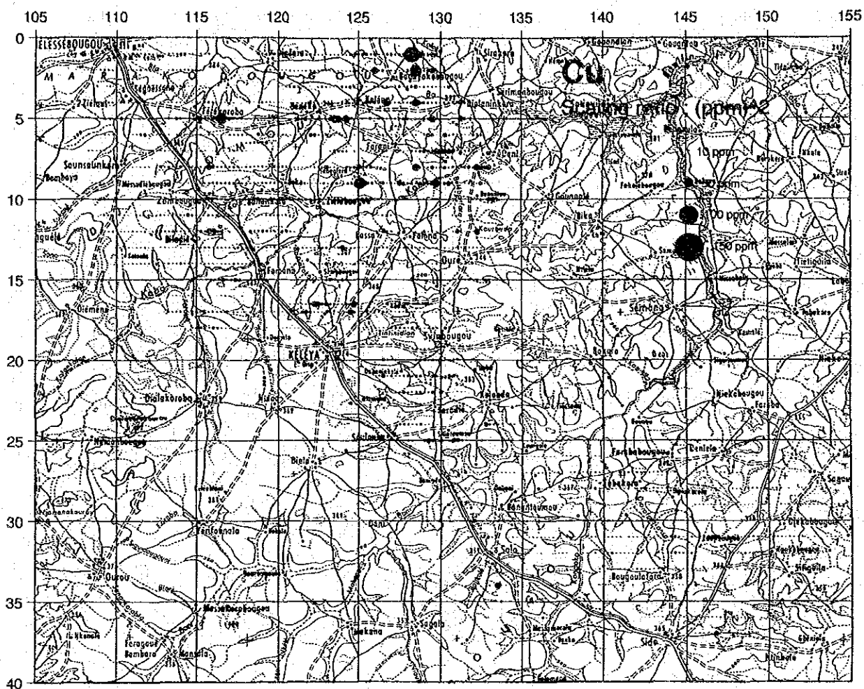
図 66 ケレヤ地区地化学探査結果図 (Cu)
