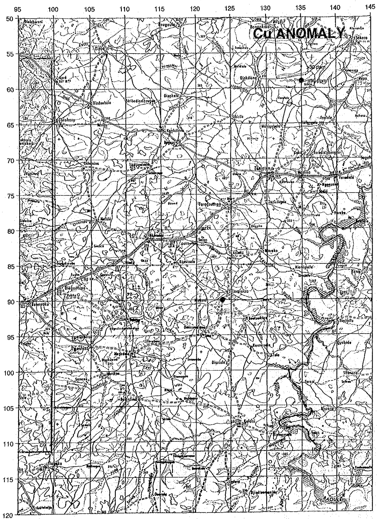
図 55 ドゥスディアナ地区地化学探査解析結果図 (Cu)
