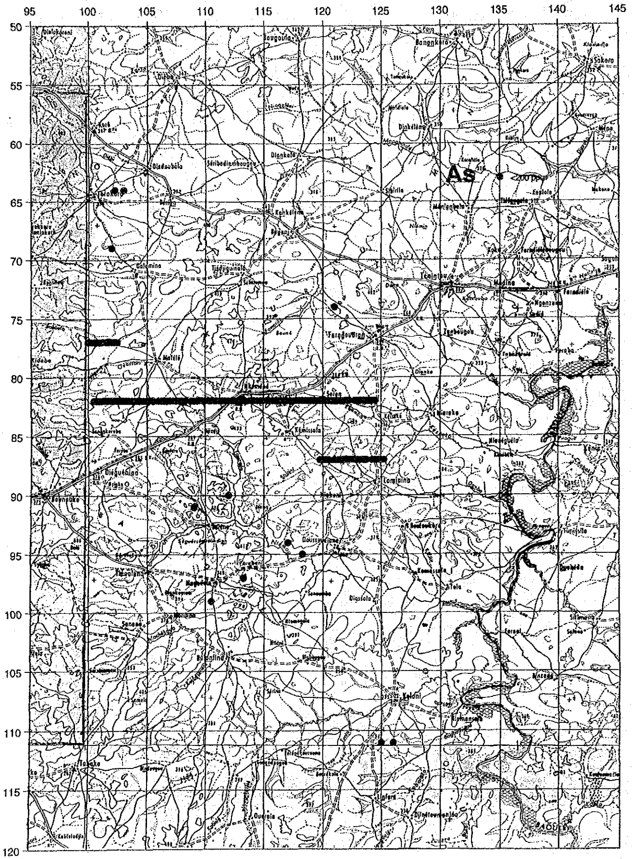
図 61 ドゥスディアナ地区地化学探査解析結果図 (As)
