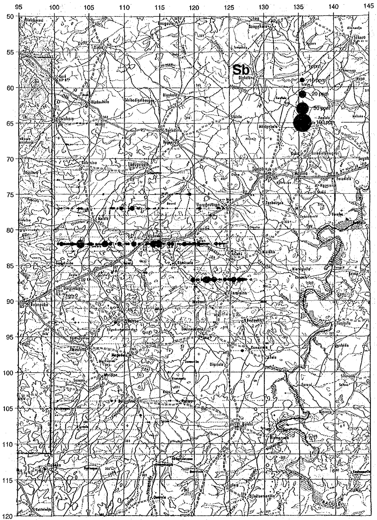
図 62 ドゥスディアナ地区地化学探査結果図 (Sb)
