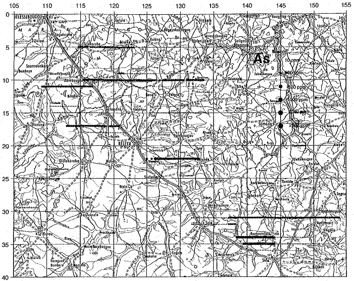
図 72 ケレヤ地区地化学探査結果図 (As)
