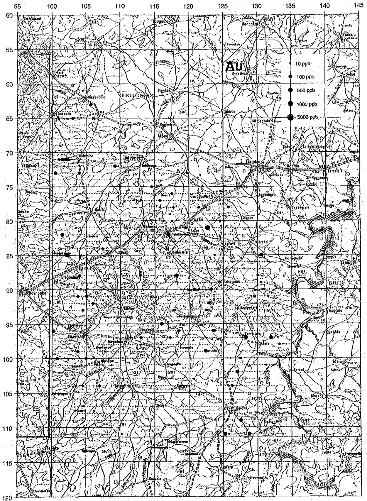
図 52 ドゥスディアナ地区地化学探査結果図 (Au)
