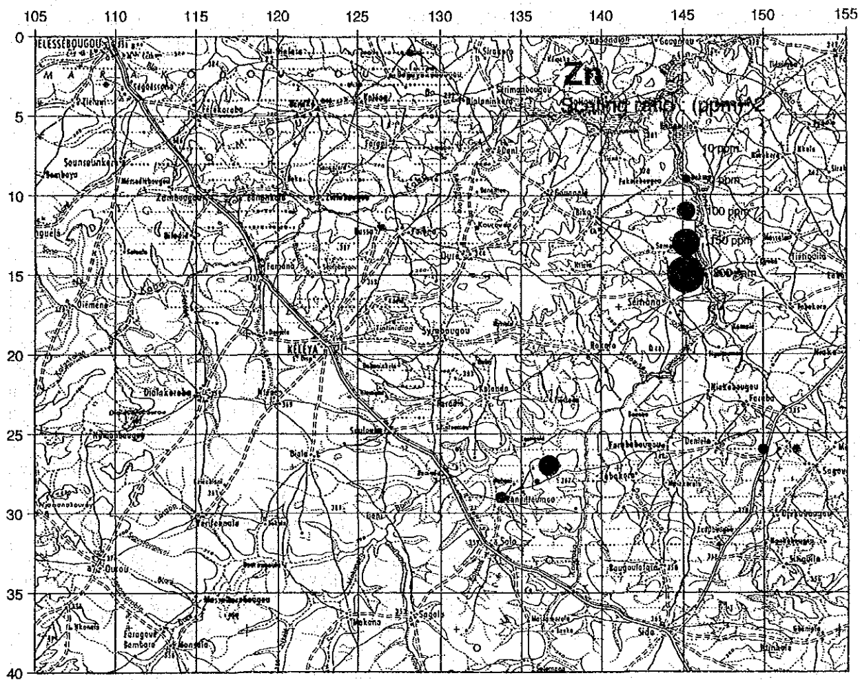
図 70 ケレヤ地区地化学探査結果図 (Zn)
