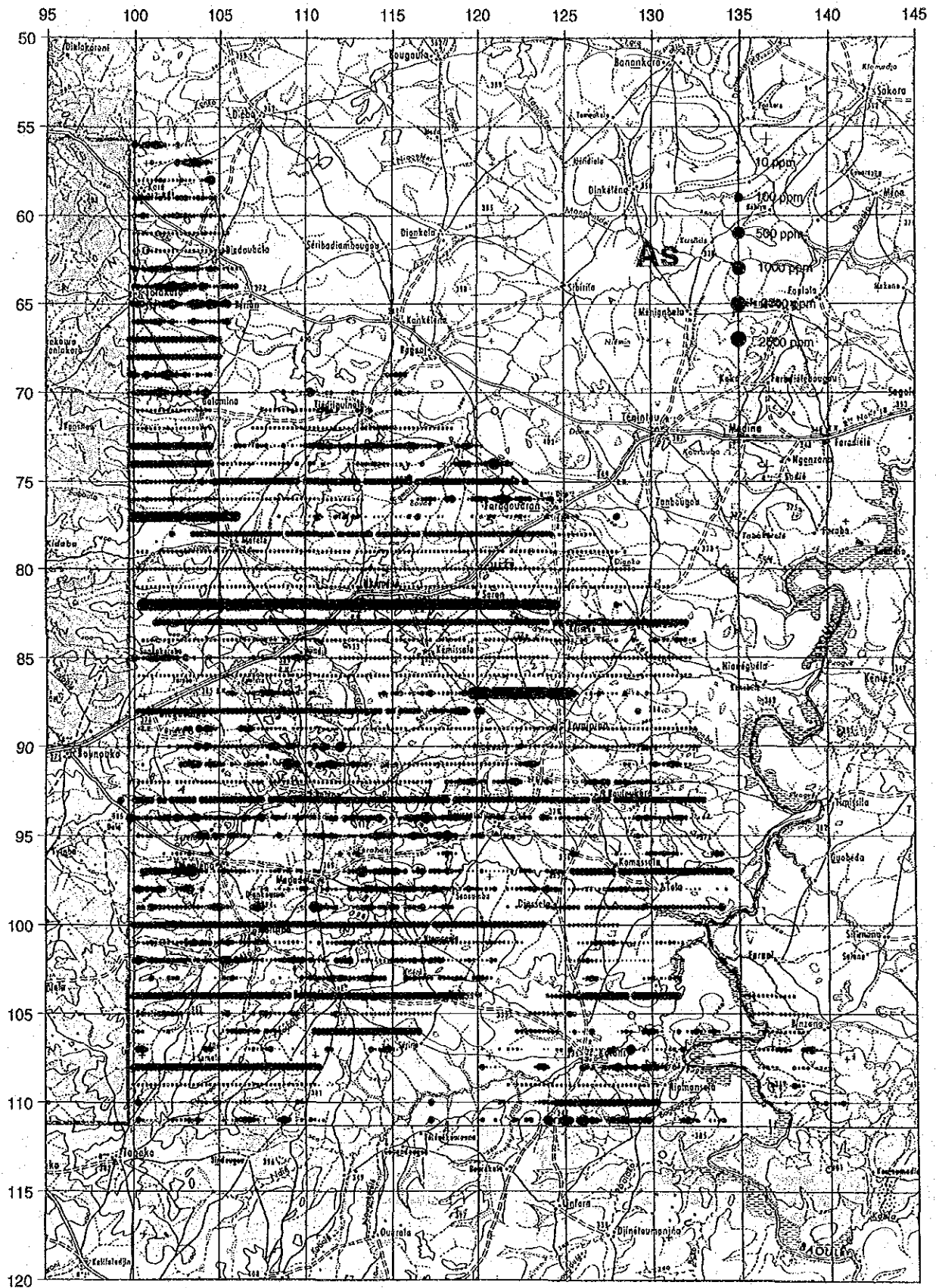
図 60 ドゥスディアナ地区地化学探査結果図 (As)
