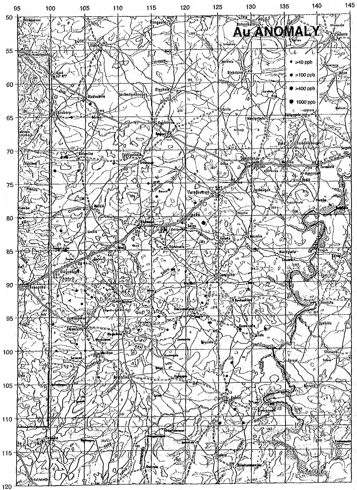
図 53 ドゥスディアナ地区地化学探査解析結果図 (Au)
