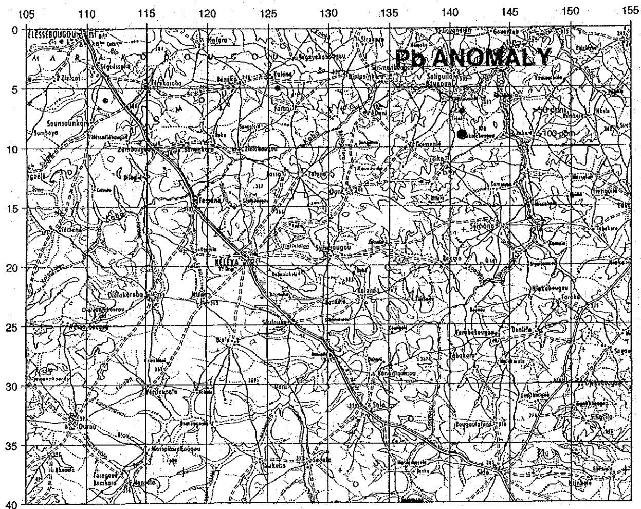
図 69 ケレヤ地区地化学探査解析結果図 (Pb)
