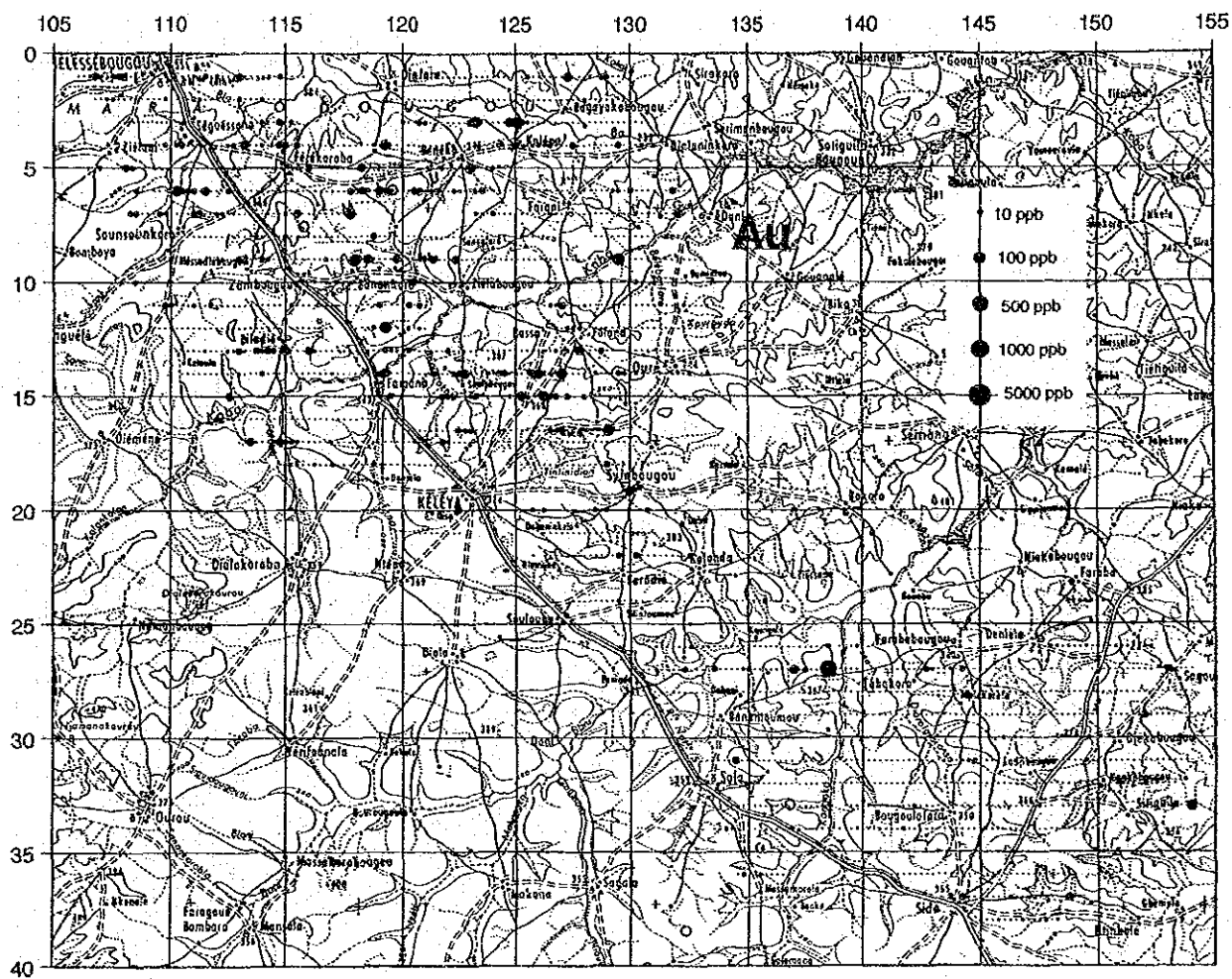
図 64 ケレヤ地区地化学探査結果図 (Au)
