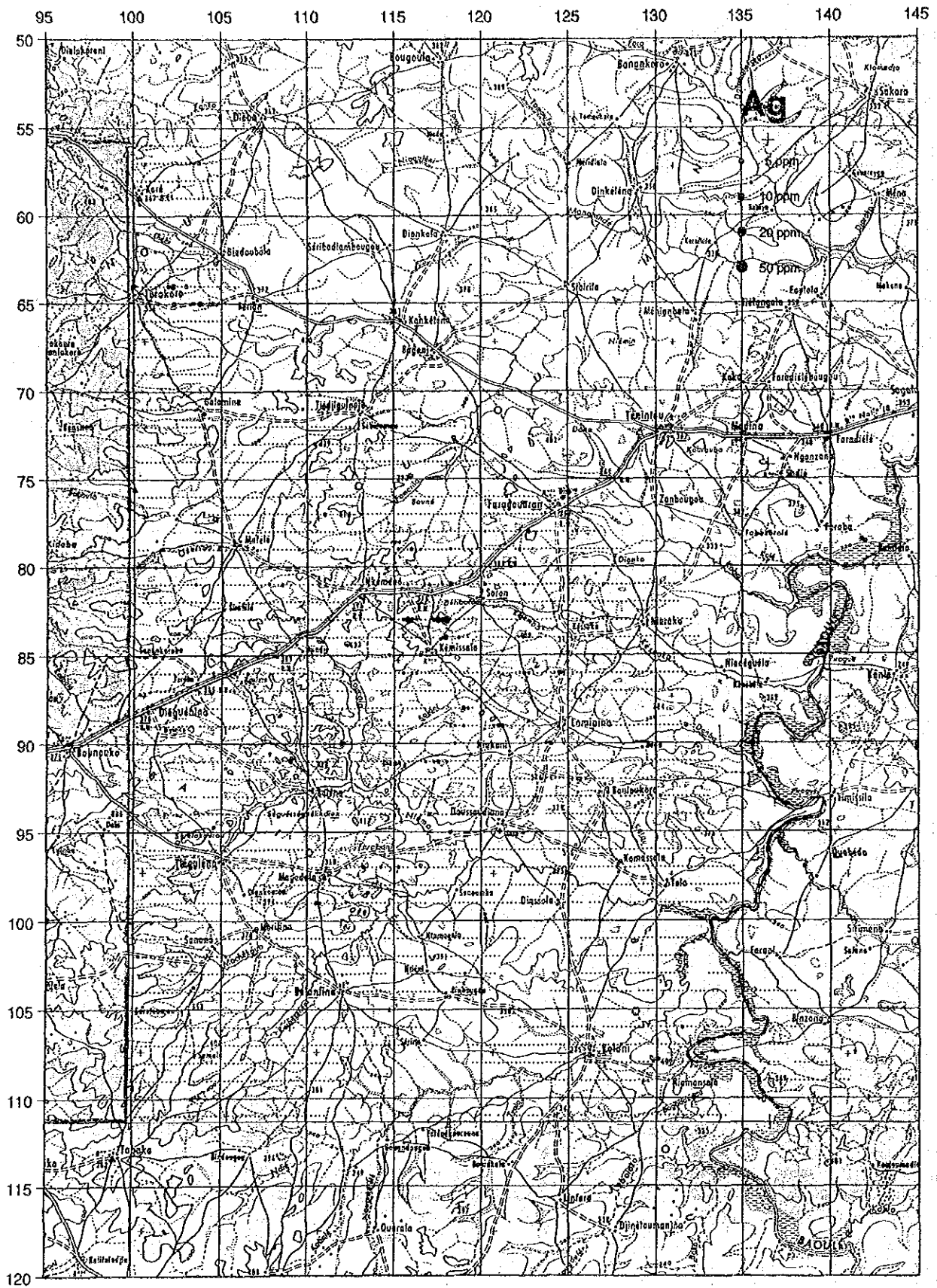
図 63 ドゥスディアナ地区地化学探査結果図 (Ag)
