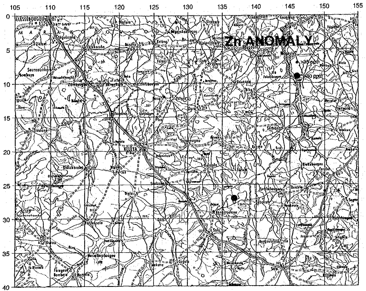
図 71 ケレヤ地区地化学探査解析結果図 (Zn)
