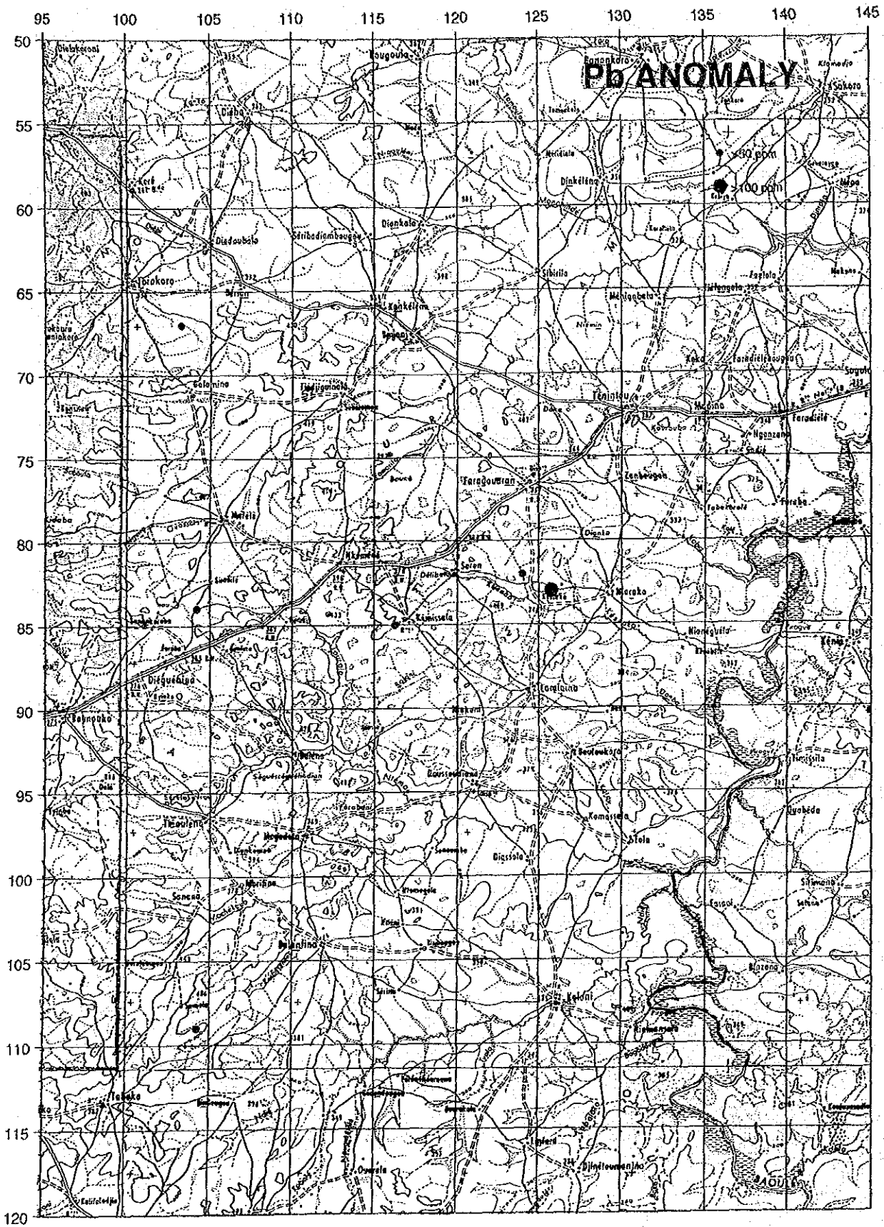
図 57 ドゥスディアナ地区地化学探査解析結果図 (Pb)
