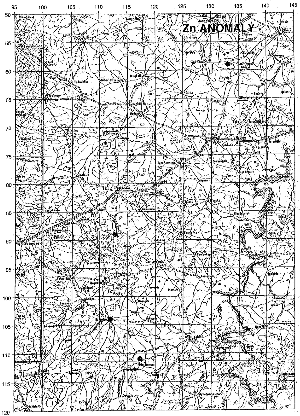
图 59 ドゥスディアナ地区地化学探査解析結果図 (Zn)
