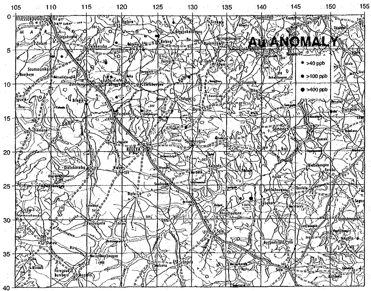
図 65 ケレヤ地区地化学探査解析結果図 (Au)
