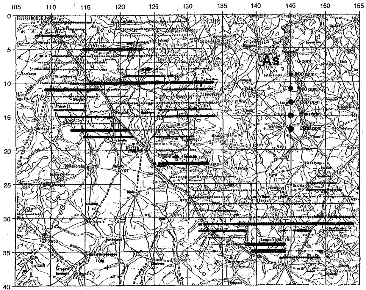
図 73 ケレヤ地区地化学探査解析結果図 (As)
