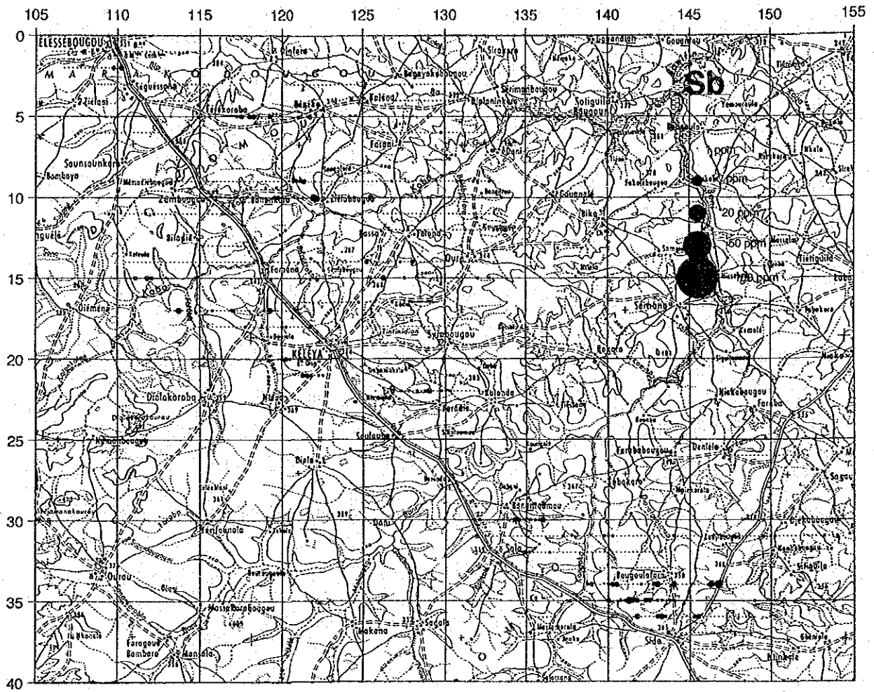
図 74 ケレヤ地区地化学探査結果図 (Sb)
