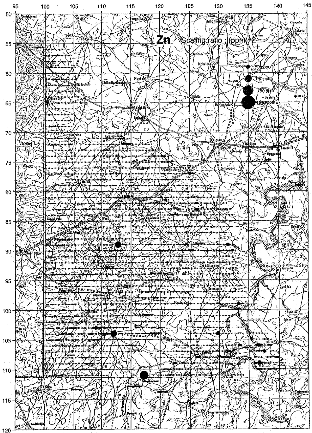
図 58 ドゥスディアナ地区地化学探査結果図 (Zn)
