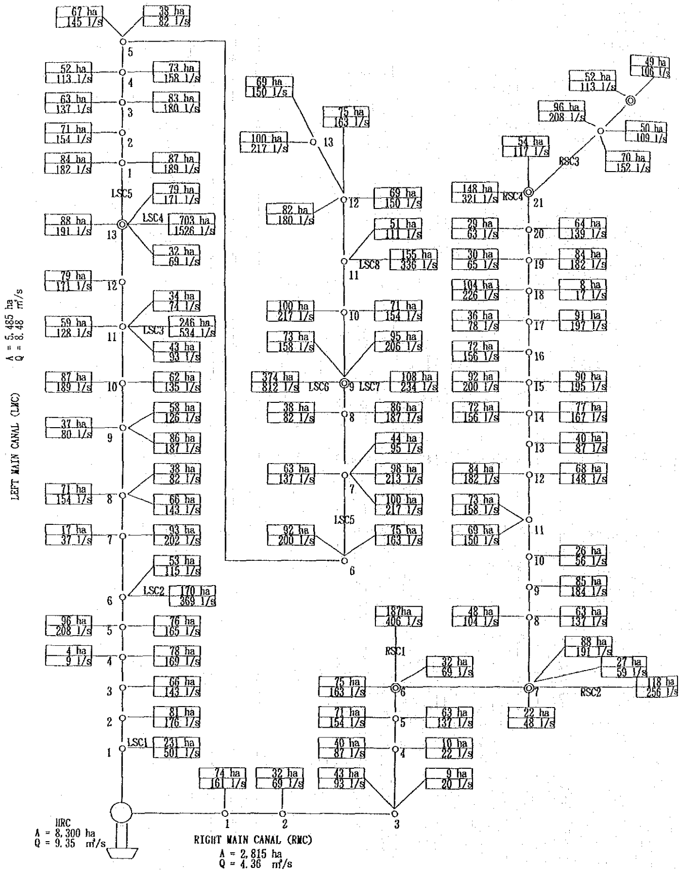
图 7.2.7 用水系統圖
