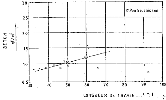
PONT A POUTRE-CAISSON EN BETON PRECONTRAIN (Quantité de béton par m 2 de la superficie de pont)
