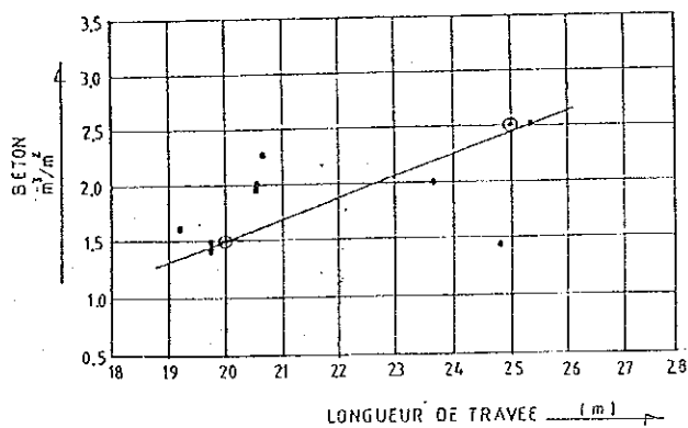
PONT A TABLIER EN DALLE ÉLÉGIE DE BETON PRECONTRAIN (Quantité de coffrage par m 2 de la superficie de pont)
