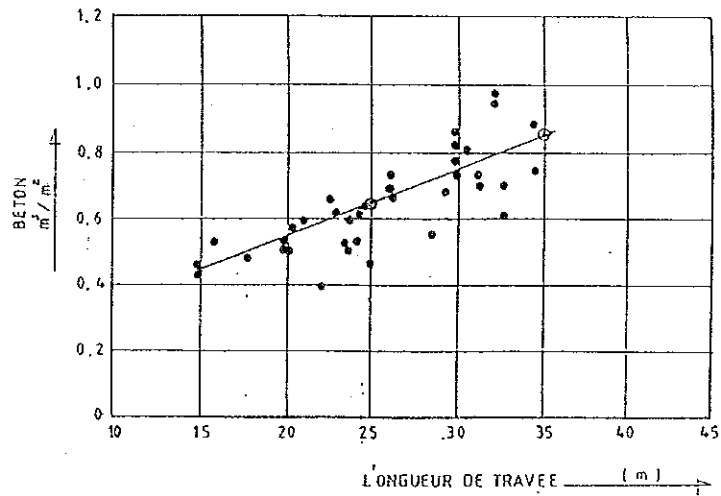
PONT A POUTRE EN T DE BETON PRECONTRAIN (Quantité de béton par m 2 de la superficie de pont)
