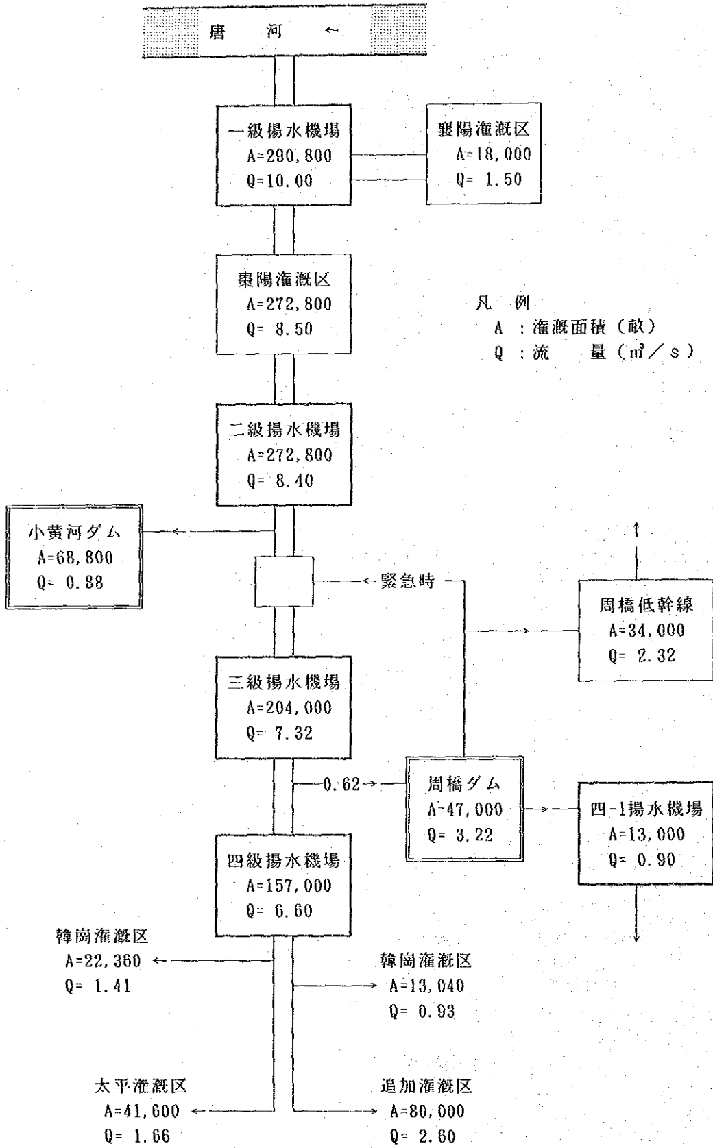
図5-2 石台寺用水系統図 (Q=10.00 m 3 /s)
