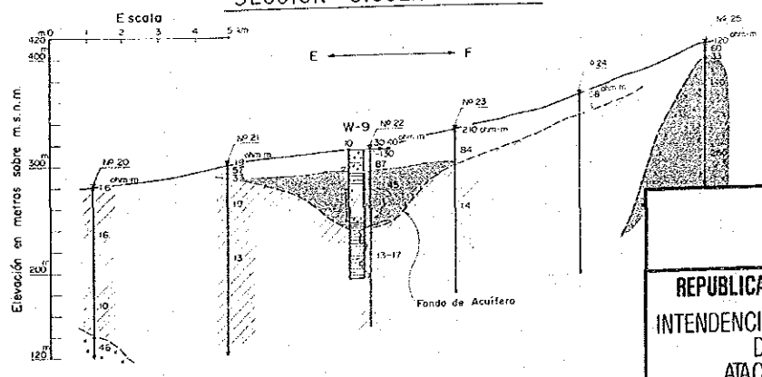
SECCIÓN SIGUENTE E - F
