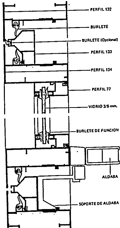
DETALLE ① CORTE VERTICAL
