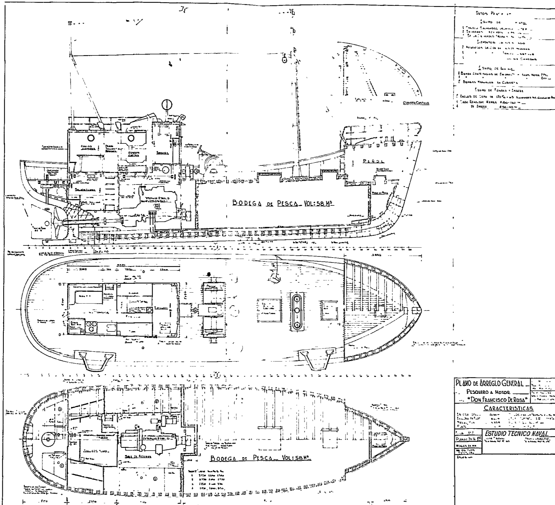
図-21 RAWSON. P・S社所属沿岸船図面 (この図面はM/P社の姉妹船図面)
