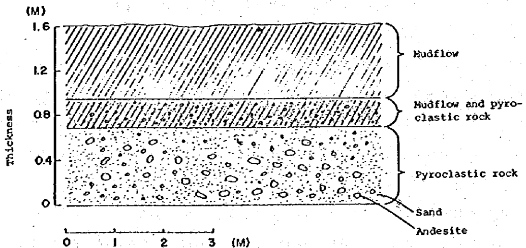
泥流の露頭
