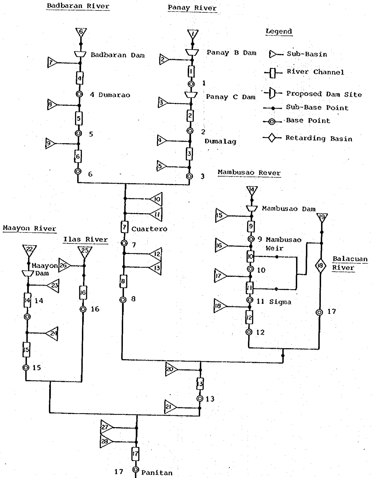
Fig. 3.5-4 RIVER SYSTEM MODEL 3.5-4 河川システムのモデル
