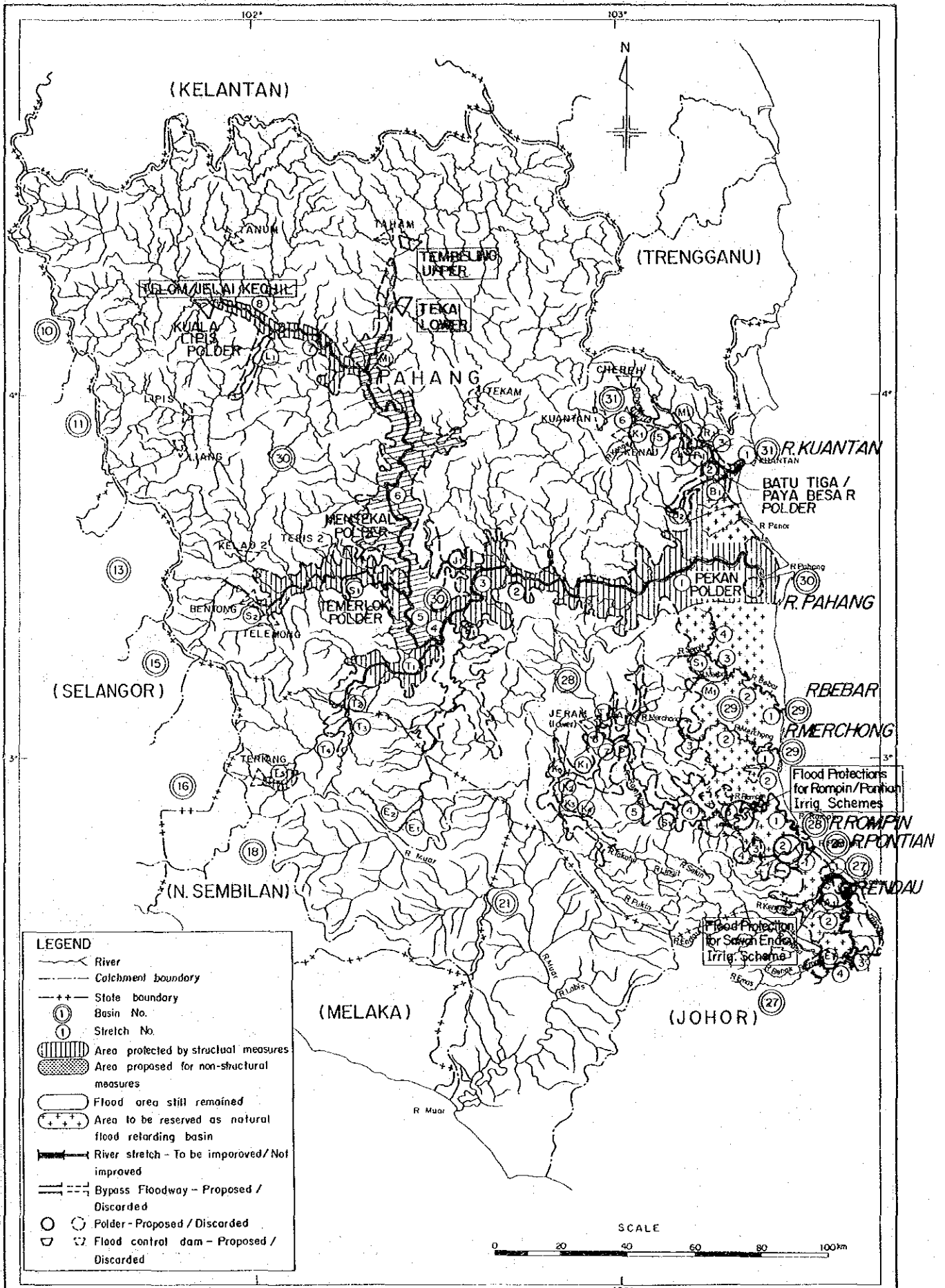
Fig. 8 Flood Mitigation Alternatives, Alternative F1
