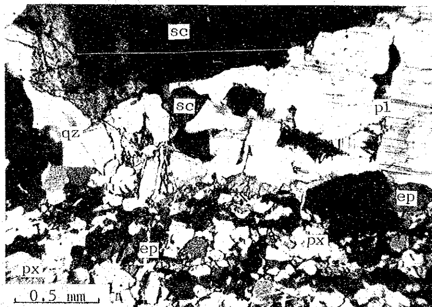
8. 含タングステン緑簾石-輝石スカルン (B-5-11) : sc; 灰重石, ep; 緑簾石, px; 輝石 (透輝石), pl; 斜長石, qz; 石英; 透過光, クロスニコル。
