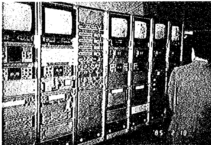
MASTER CONTROL ROOM機器室 (此処でPAL/SECAM変換を行っている)
