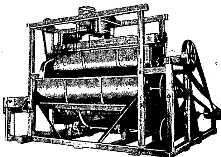
名称 BRILHADOR DE ARROZ 白米研磨機
