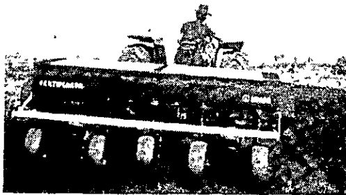
名称 FERTIPLANTA DE ARRASTRO 施肥植付機
