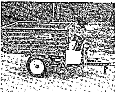
とくにコーヒー國 用畜糞散布機
