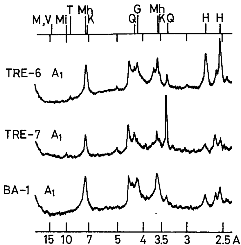
図-6 TRE及びBAの粘土部分のX線回折像：K,カオリナイト；Mh,メタハロイサイト；Mi,雲母鉱物；M,V,モンモリロナイト又はバーミキュライト；T,タルク；G,ゲータイト；H,ヘマタイト；Q,石英。
