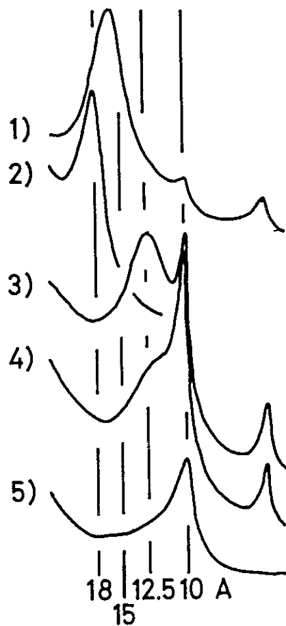
図-5 GPH-1のCg層(21142)における(001)回折ピークの変化: 1) Mg^{2+} 飽和, 室温 2) Mg^{2+} 及びグリセロール飽和 3) K^+ 飽和, 室温 4) K^+ 飽和, 300°C加熱 5) K^+ 飽和, 600°C加熱。
