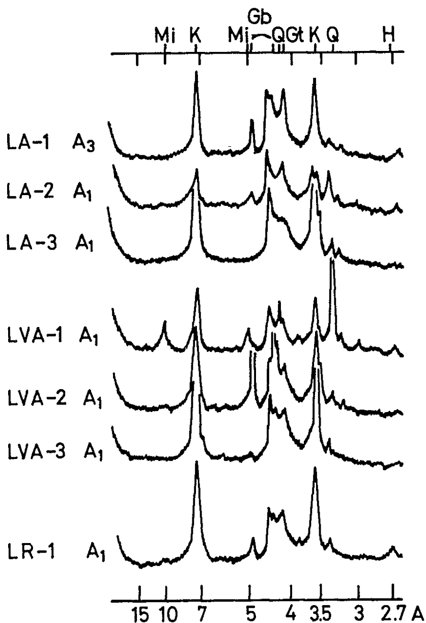
図-2 オキシックB層をもつ土壤の粘土部分のX線回折像：K，カオリナイト；Mi，雲母鉱物；Gb，ギブサイド；Gt，ゲータイト；H，ヘマタイト；Q，石英。
