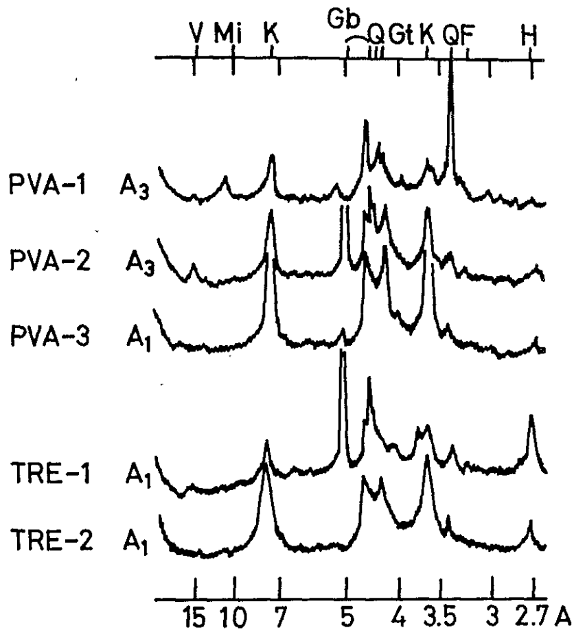
図-3 土性B層をもつ土壤の粘土部分のX線回折像：K，カオリナイト；Mi，雲母鉱物；V，パーミキュライト；Gb，ギブサイト；Gt，ゲータイト；H，ヘマタイト；Q，石英；F，長石。
