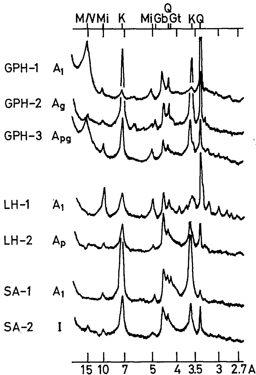
図-4 低地土壌の粘土部分のX線回折像：K, カオリナイト；Mi, 雲母鉱物；M/V, モンモリロナイト/パーミキュライト混合層鉱物；Gb, ギブサイト；Q, 石英
