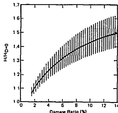
図9-1-3 被害率と波高の関係(ウーレ)
