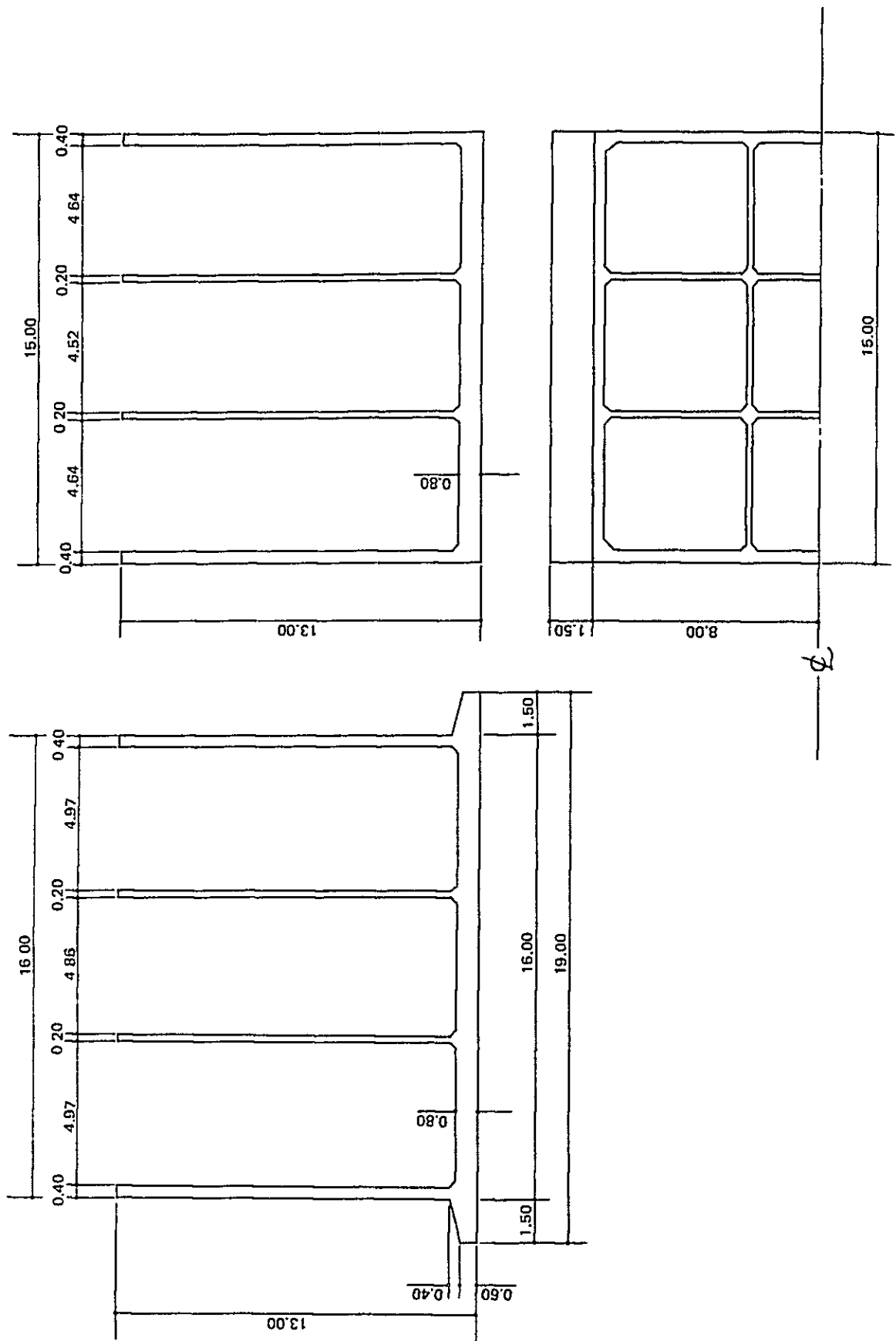
図9-1-7 ケーソン構造図
