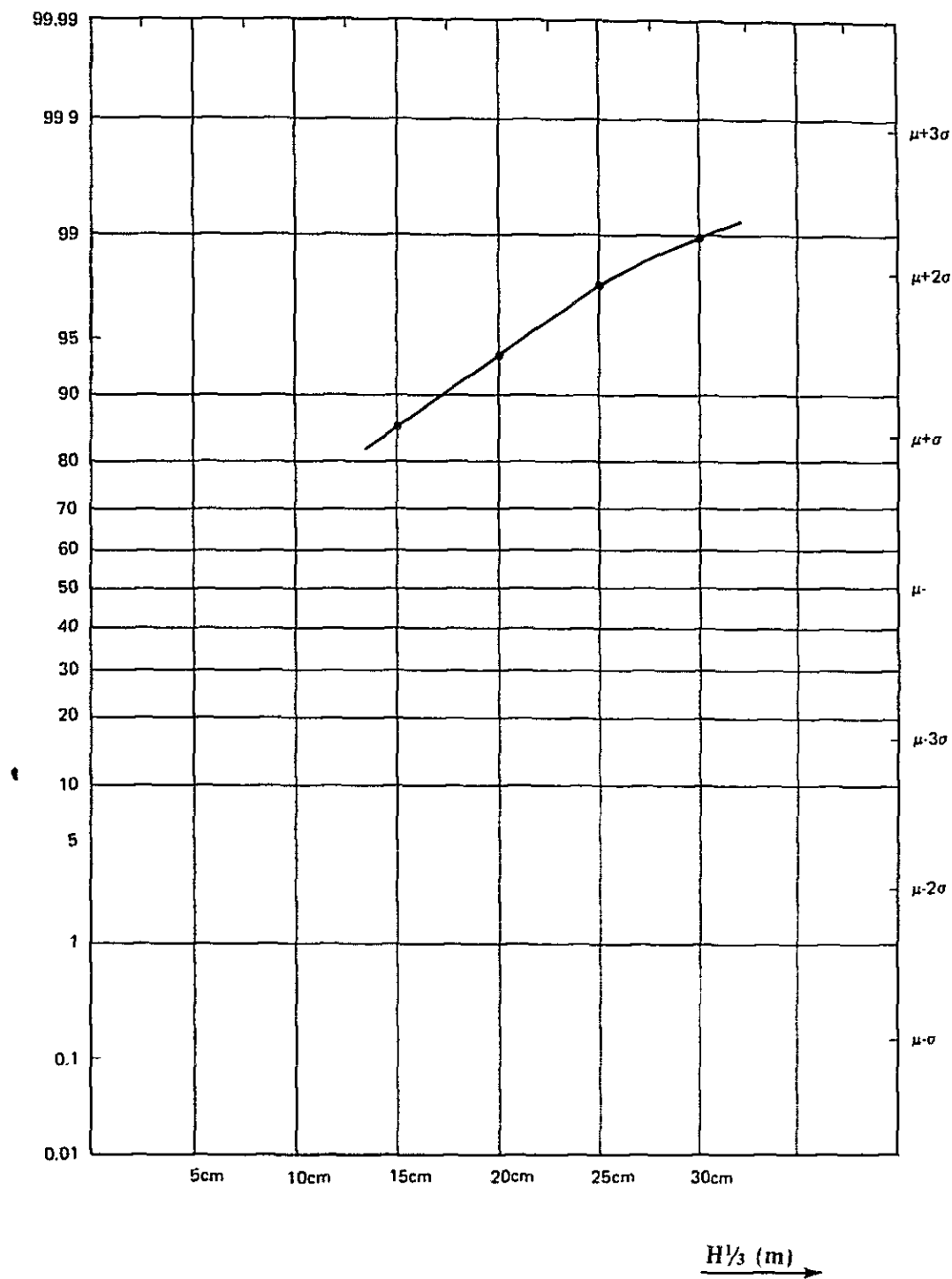
図 8-3-12 第Ⅱ期計画の埠頭前面波高の未超過確率図
