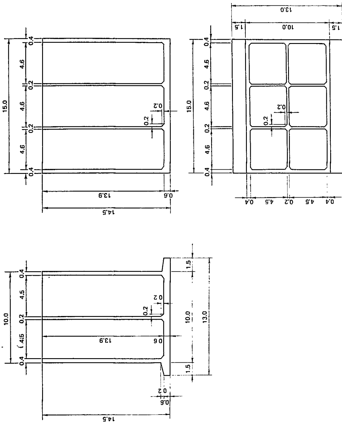
図9-1-11 ケーン構造図
