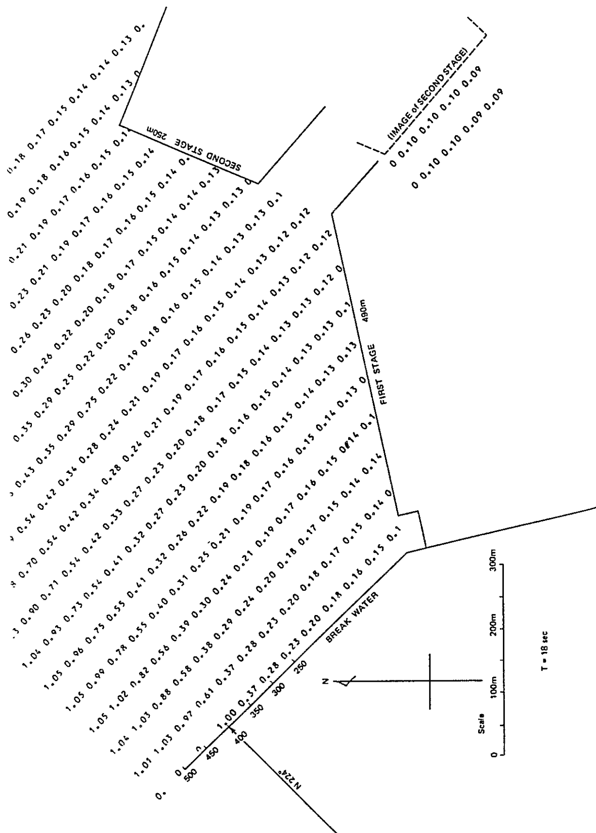
図 8-3-7 回折図(6)防波堤400m 入射波向N224° 周期18sec
