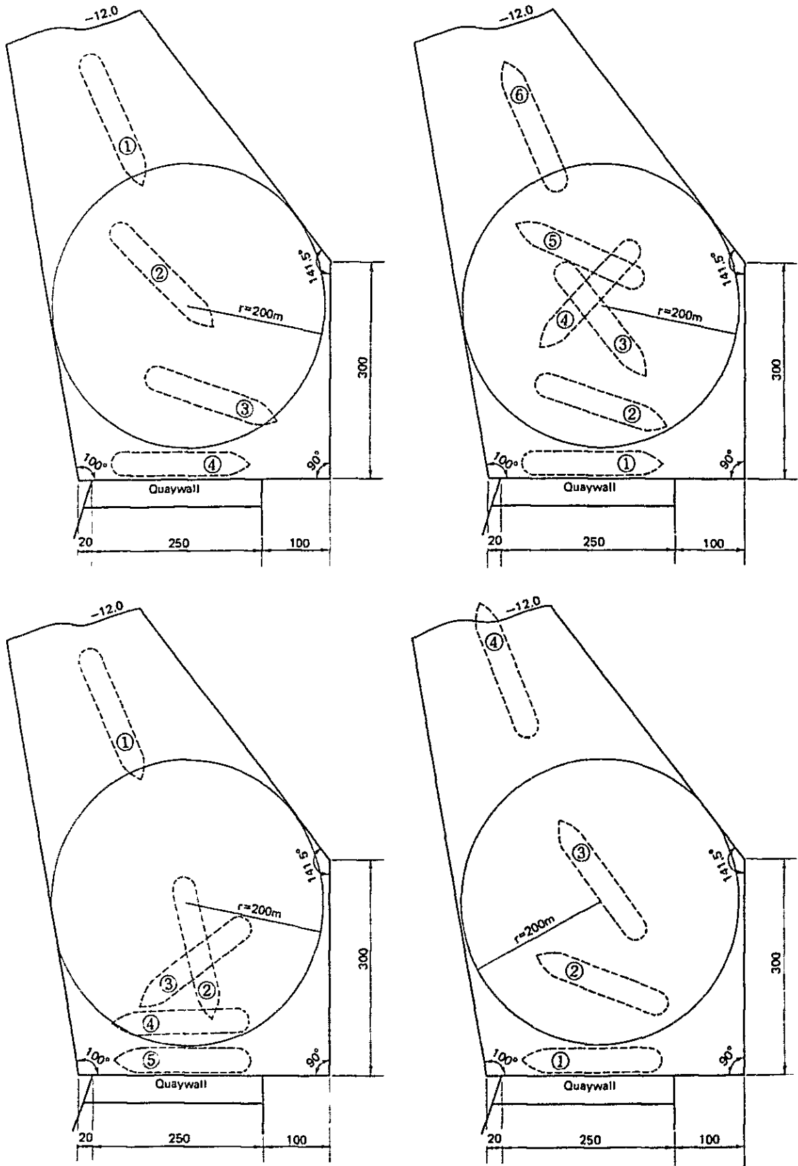
图9-1-13 泊地
