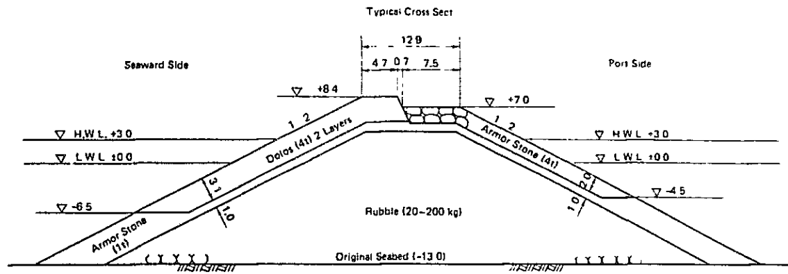
図9-1-4 消波ブロック式防波堤
