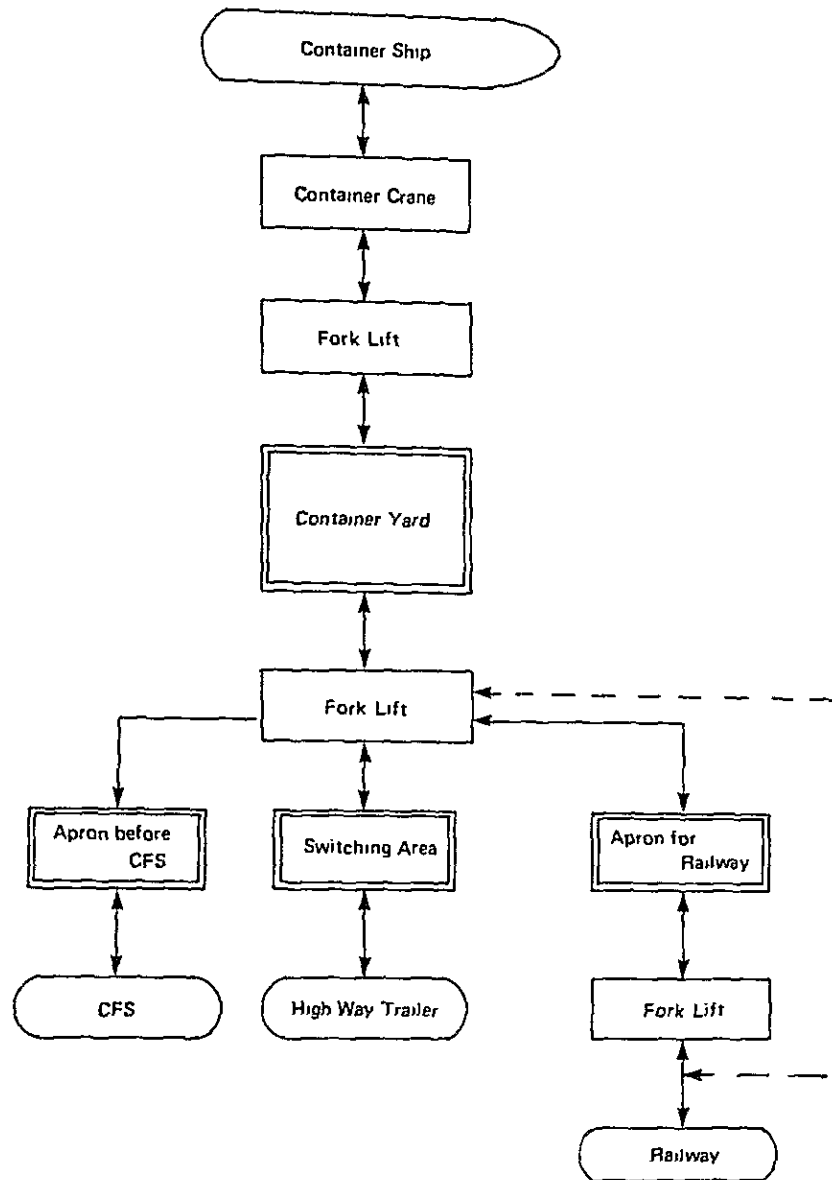
図 8-2-4 フォークリフトシステム
