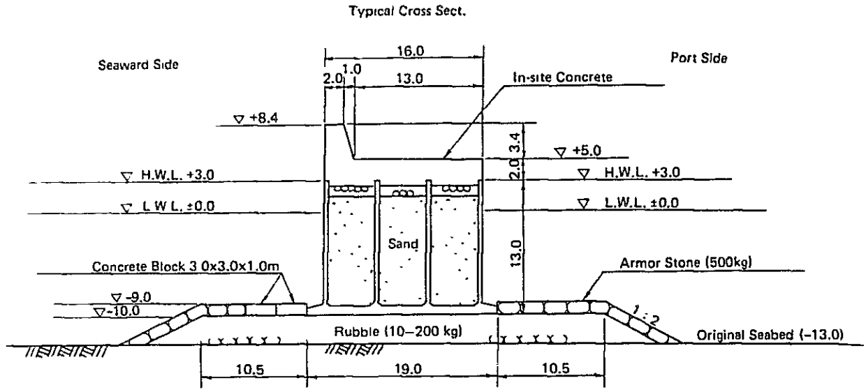
図9-1-5 ケーソン式防波堤
