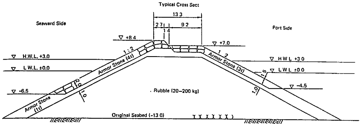
图 9-1-1 抛石式防波堤
