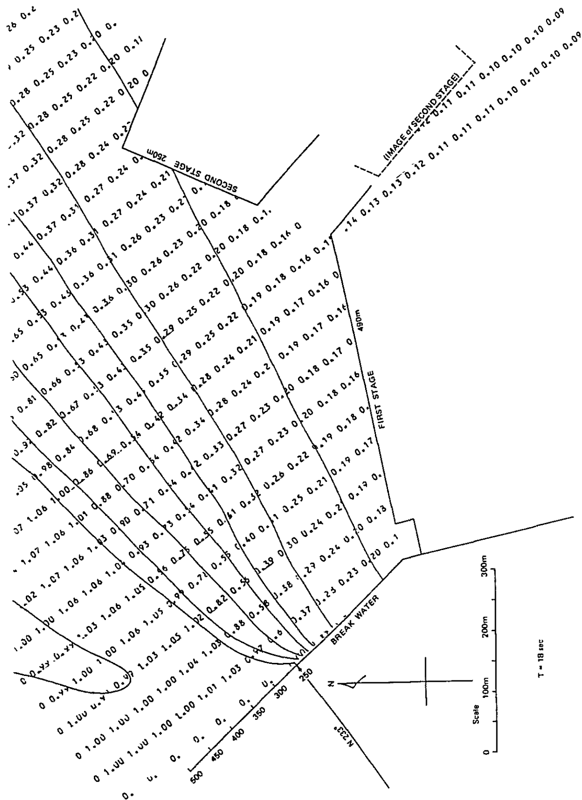
图 8-3-2 回折图(2)防波堤 250m, 周期 18sec
