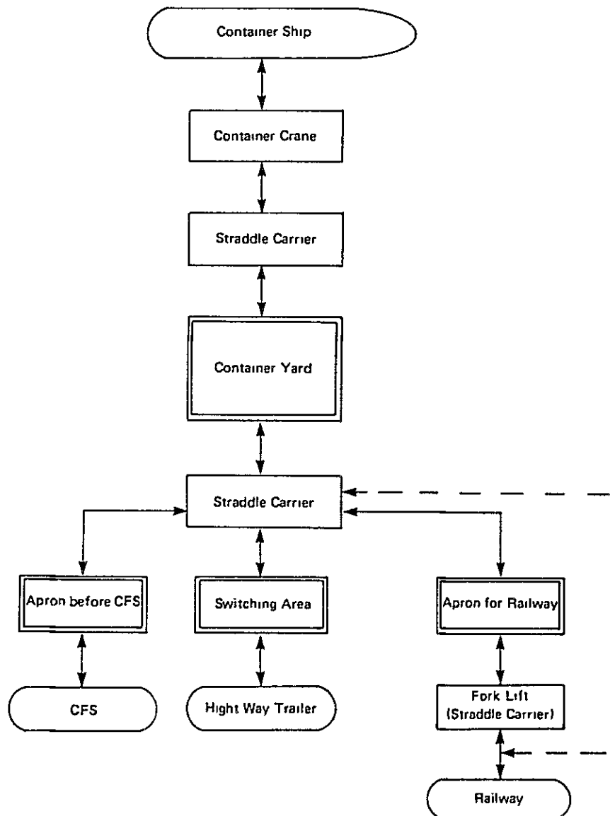
図 8-2-3 ストラドルキャリアシステム
