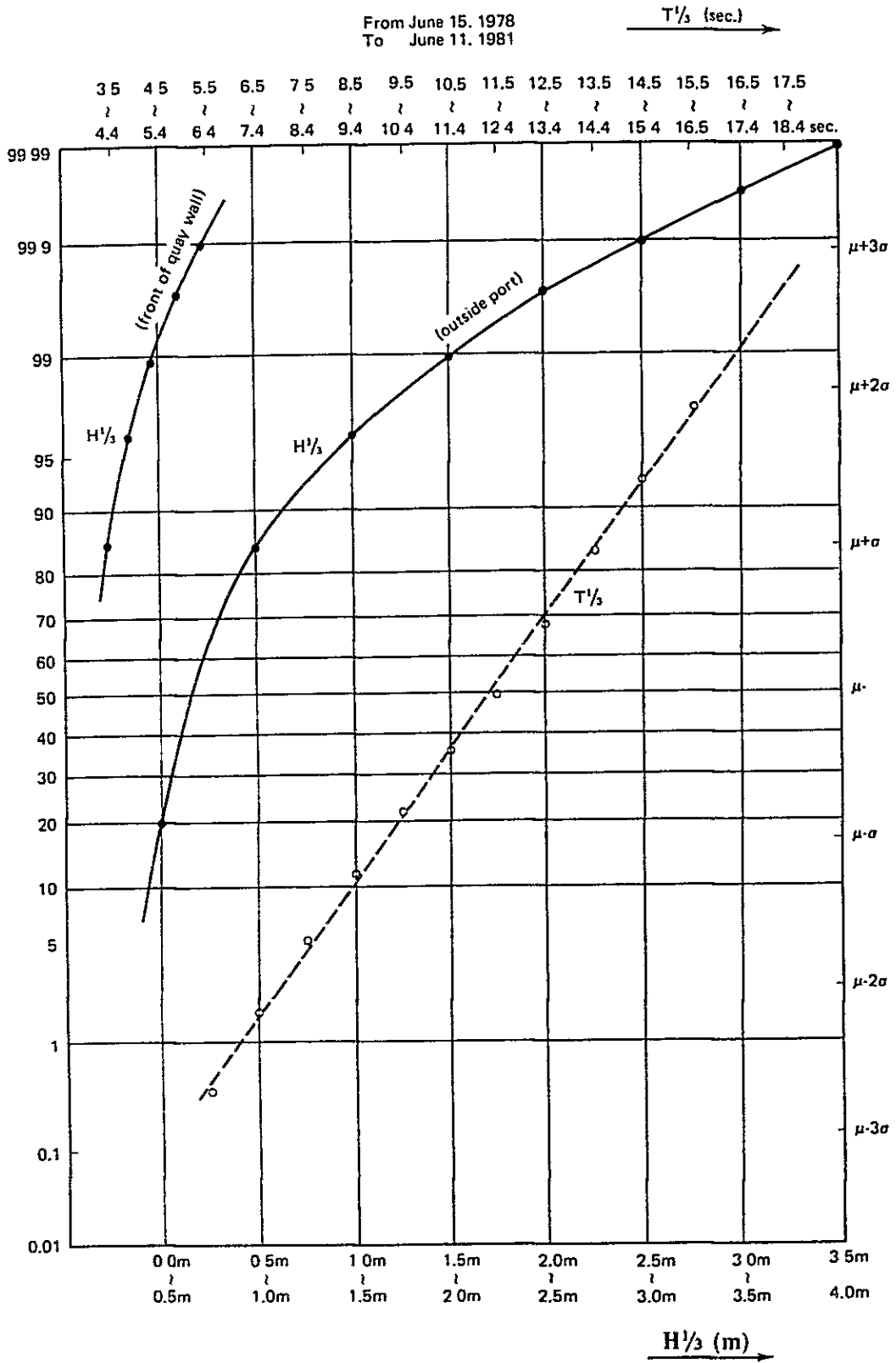
圖 8-3-3 波高出現未超過確率
