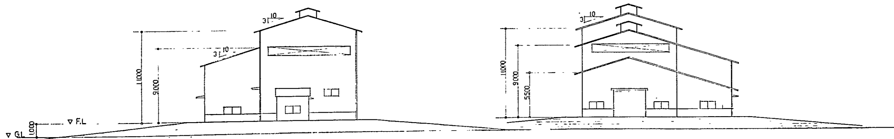
ライス・ミル建物 (150トン/日産ライス・ミル) バセイン, カナントー Fig. 19 BUILDING FOR RICE MILL PLANT BASSEIN & KANAUNGTOE (150 TONS PER DAY RICE MILL)
