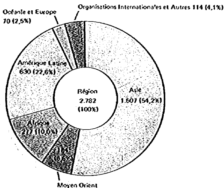
Fig. 2 Nombre Total des Experts Envoyés par Secteur et par Région (1955-1984)
