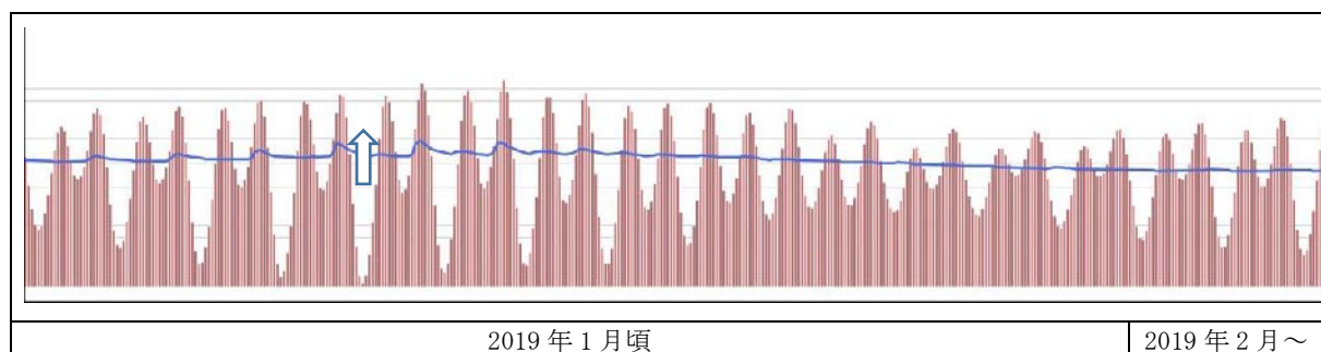
図 4.3.3.4 潮位と地下水位の関係（時間最大値）
