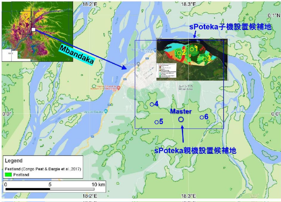
図 5.1.2.2 赤道州 Mbandaka 近郊 Jardin Botanique d' EALA 泥炭湿地位置図
