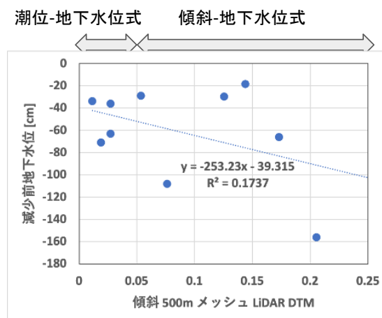
図 4.3.3.6 LiDAR の標高から計算された傾斜と、BRG 観測所から得られた無降水期間が開始する前日の地下水位の関係
