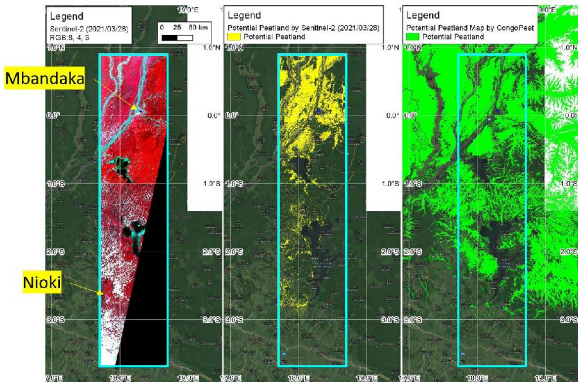
図 3.2.1.12 2021 年 3 月 28 日に観測された Sentienl-2 画像を用いた泥炭地抽出結果
