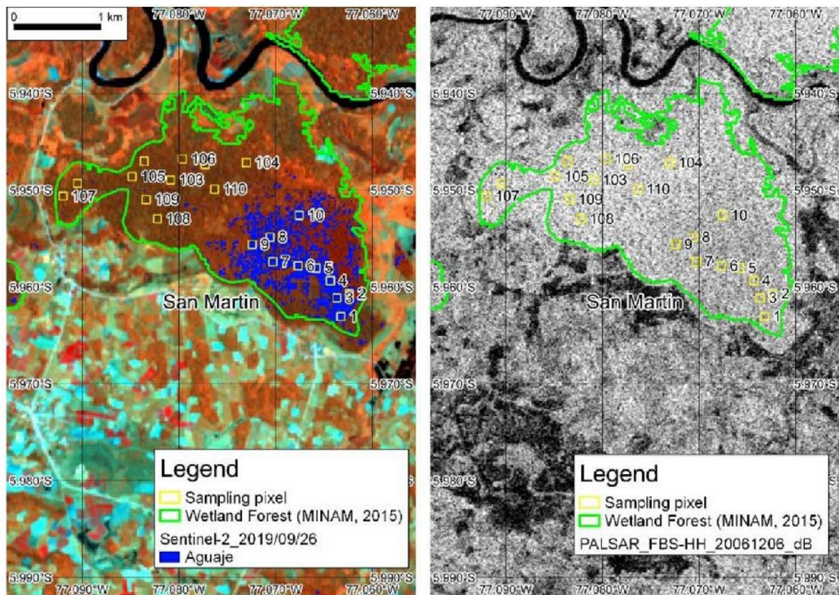
図 3.2.4.1 Yantaro 北西地区の Sentinel-2（左）と PALSAR/FBS-HH（右）
