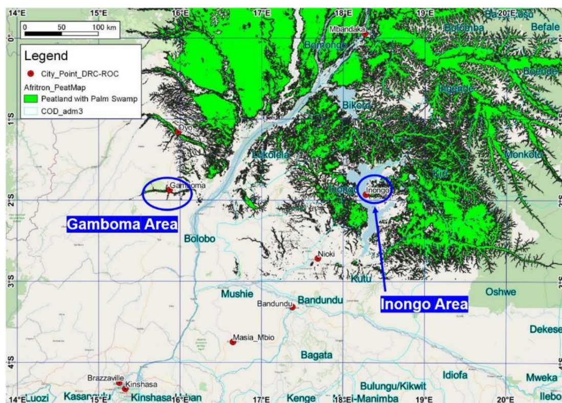
図 3.2.3.1 Gamboma 地区及び Inongo 地区位置図
