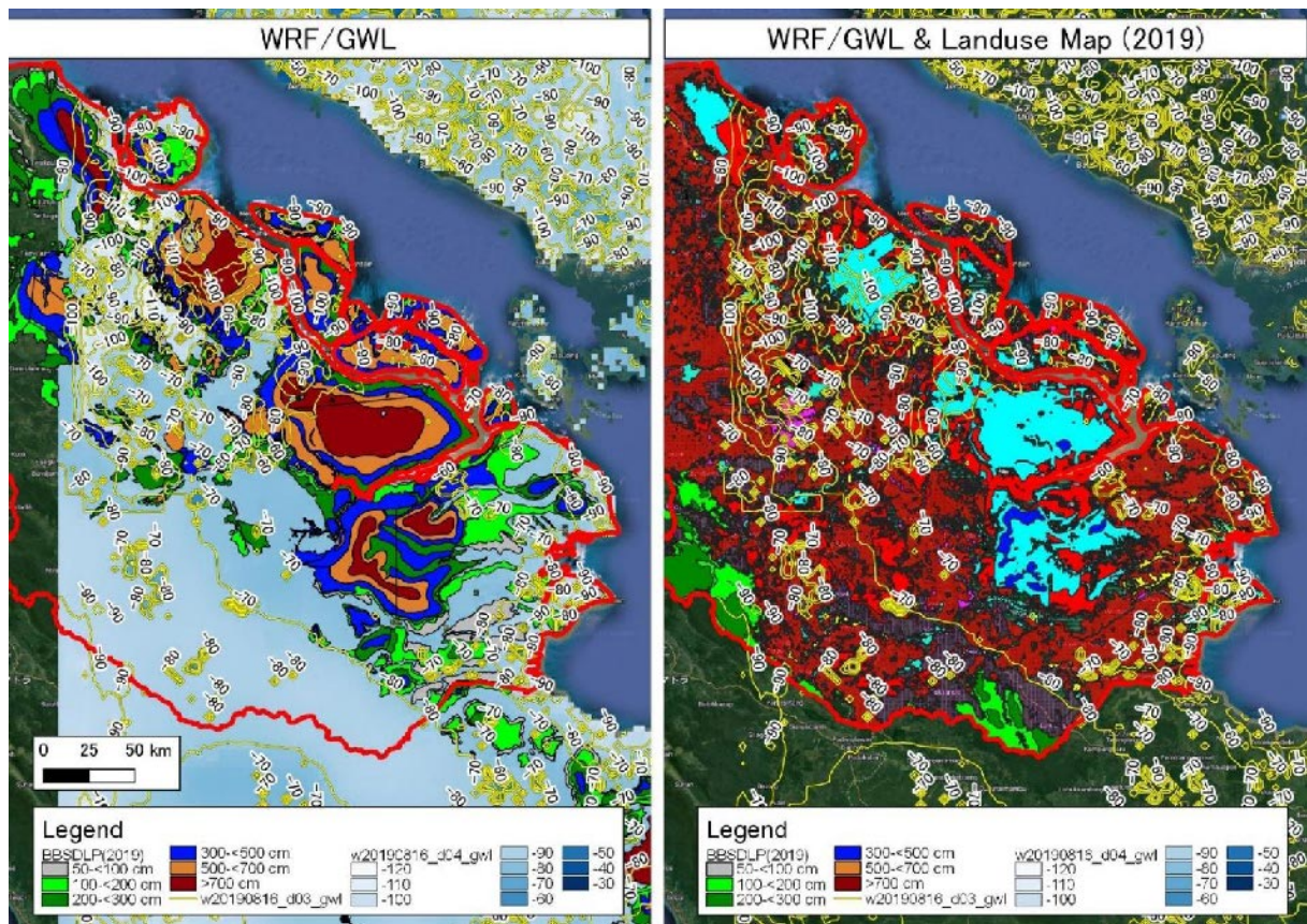
図 4.7.2.16 リアウ州における地下水位等深度線（10cm 単位）、BBSDLP 泥炭図及び土地被覆図（2019）
