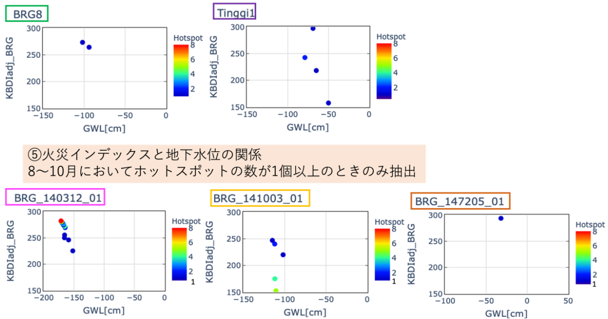
図 4.6.4.1 5つのBRG観測所データから計算された火災インデックス（KBDIadj）と地下水位日最大の散布図
