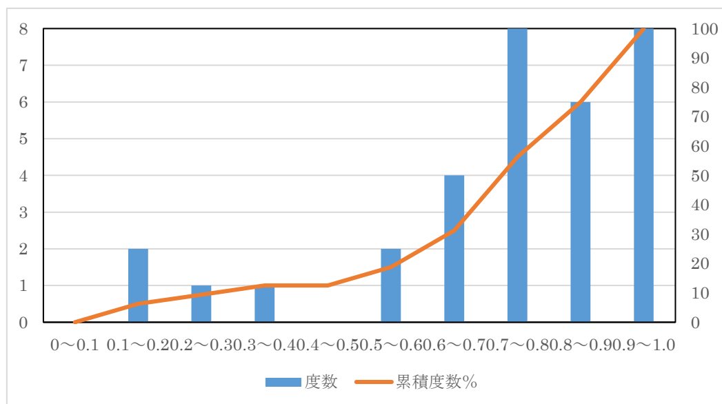
図 4.2.1.6 WRF を用いたシミュレーションによる地下水位推定の絶対係数
