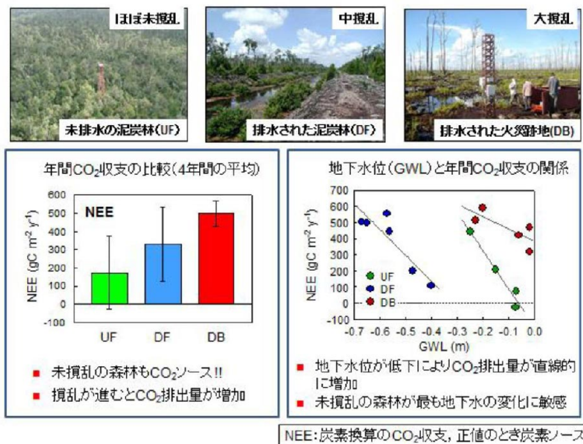
図 5.1.1.2 年間 \text{CO}_2 収支の比較、地下水位（GWL）と年間 \text{CO}_2 収支の関係 85
