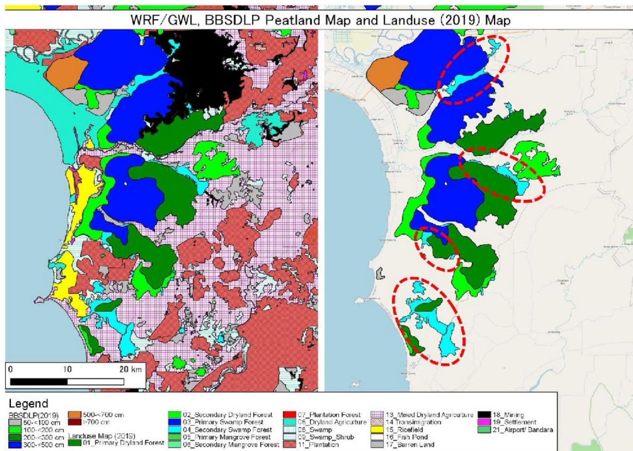
図 4.7.2.13 西カリマンタンにおける地下水位等深度線（-75cm）、BBSDLP 泥炭図による泥炭マッピング結果
