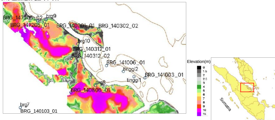
BRG 観測所全16地点 リアウ州
