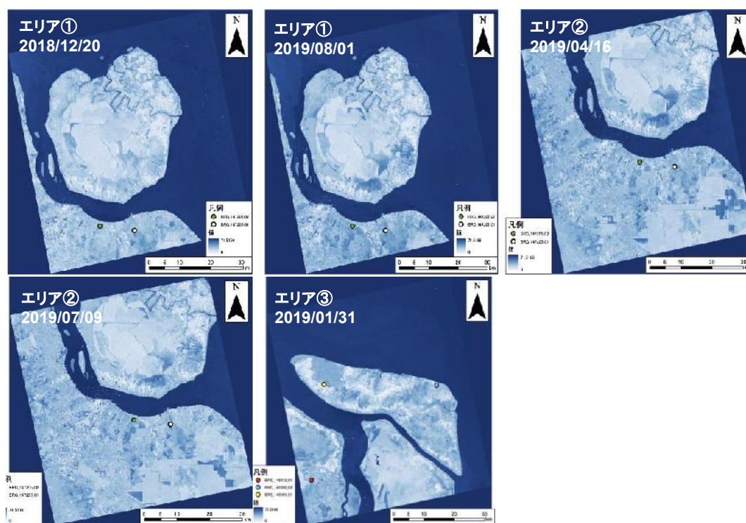
図 4.2.2.2 すべてのエリアを合わせた場合の土壌水分量の推定結果
