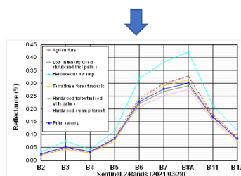
図 3.2.1.9 大気補正済及び大気補正未処理 Sentinel-2 画像における泥炭地植生のスペクトル特性
