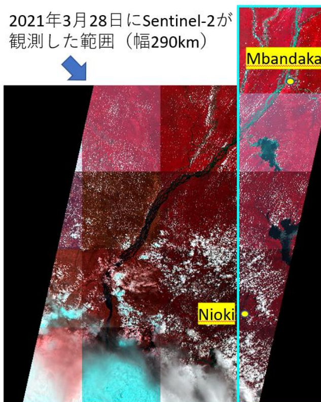
図 3.2.1.11 Mbandaka から Nioki を含む 2021 年 3 月 28 日に観測された Sentinel-2 画像
