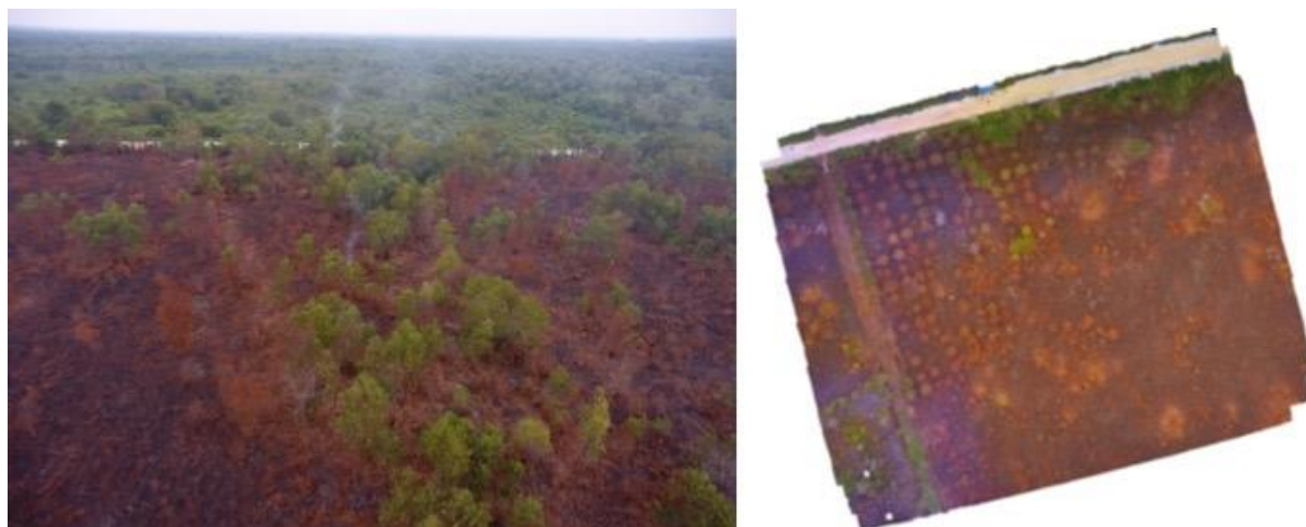
図 4.6.5.1 リアウ東部プララワンにて空撮されたドローンの可視画像及び可視カメラのオルソ画像を地図化した例（2022 年 8 月 18 日撮影）
