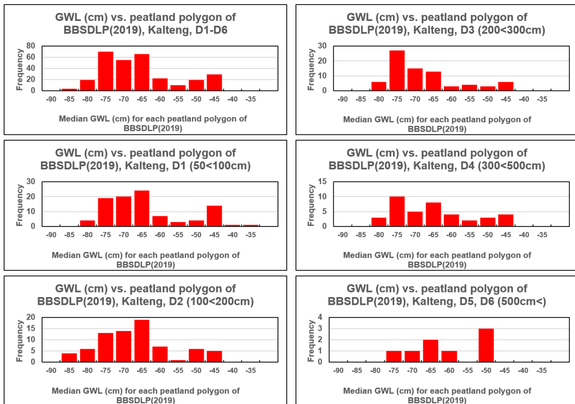
図 4.7.2.3 中央カリマンタン州 BBSDLP 泥炭図における泥炭の厚さごとの地下水位頻度分布（各泥炭図ポリゴンで 3km グリッドの WRF 地下水位値を抽出した結果）
