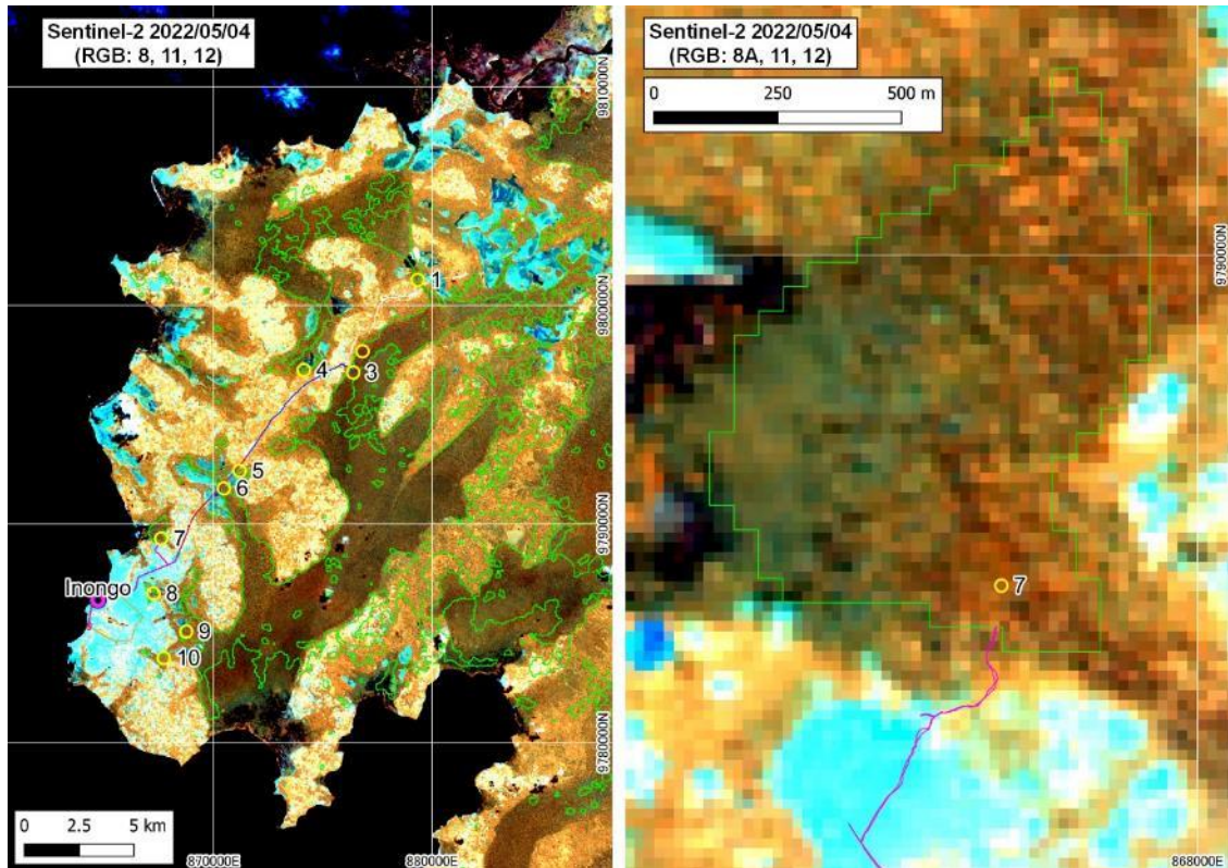
図 3.2.3.10 Inongo 地区の調査地点 (No. 7)
