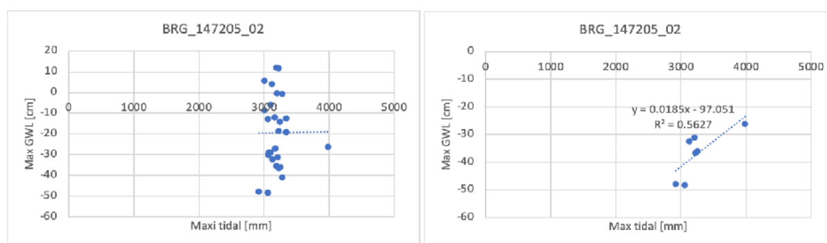
図 4.3.3.5 潮位と地下水位の散布図（それぞれ月最大値）
