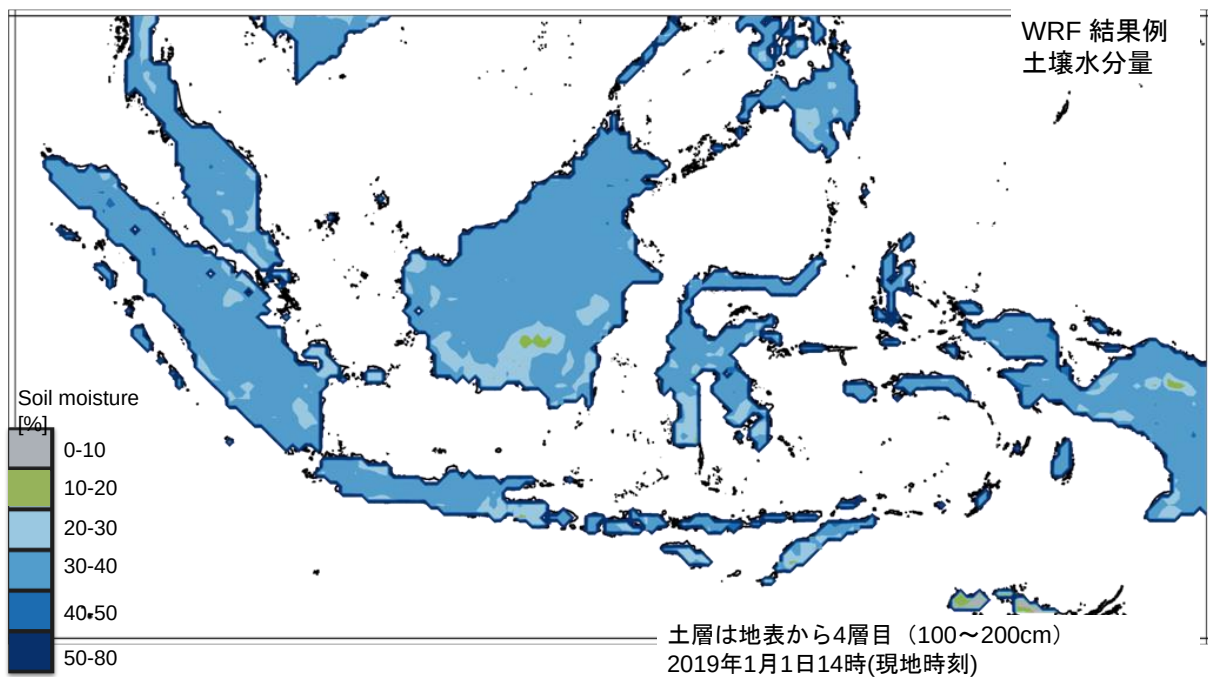
図 4.2.1.3 2019 年 1 月 1 日 14:00 (現地時間) の WRF の結果の例 (地表から 4 層目の土壌水分量)
