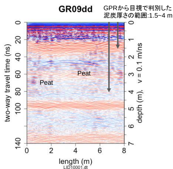
図 4.7.1.4 観測所 9(140806_01)における GPR の計測結果の例
