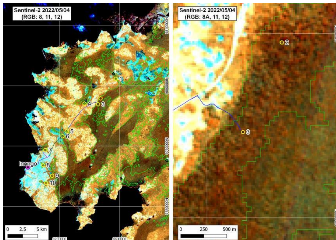
図 3. 2. 3. 5 Inongo 地区の調査地点 (No. 3)
