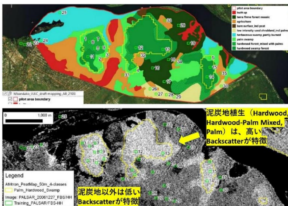
図 3.2.1.16 Mbandaka 土地被覆図と PALSAR/FBS モード画像
