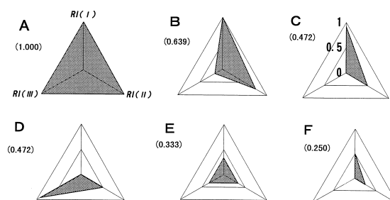
図 1 指標グループごとに求めた RI 指数のレーダーチャート
