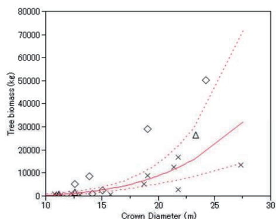
図 T17-b 樹冠径と単木バイオマスの関係 (Kiyono et al. 2) より作図)
