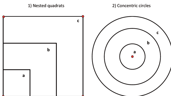
図 T13-1 プロットの形状
