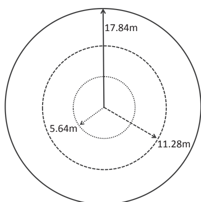
図 P10-1 4km メッシュで配置された日本の PSP におけるプロット形状
