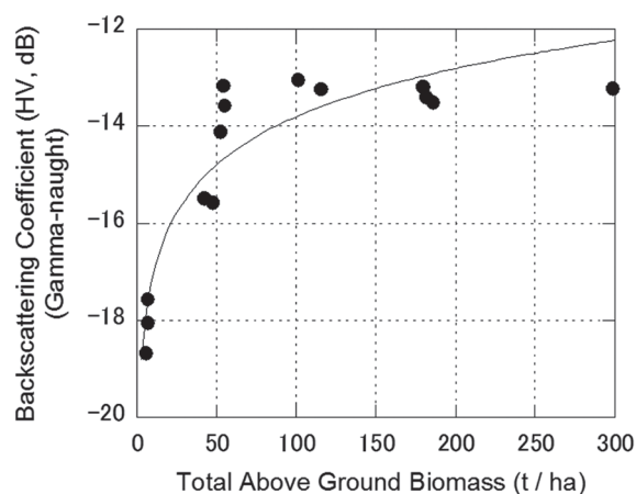
図 T19-1 後方散乱係数とバイオマスの関係
