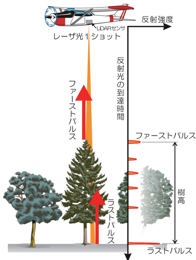
図 T05-2 LiDAR によるデータ取得の概念
