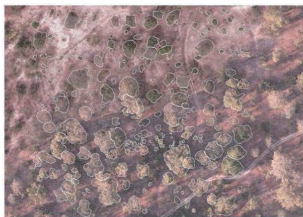
図 T17-2 デジタル空中写真の実体視計測による樹冠ポリゴンの抽出 (カンボジア、コンポントム州、乾燥フタバガキ林)
