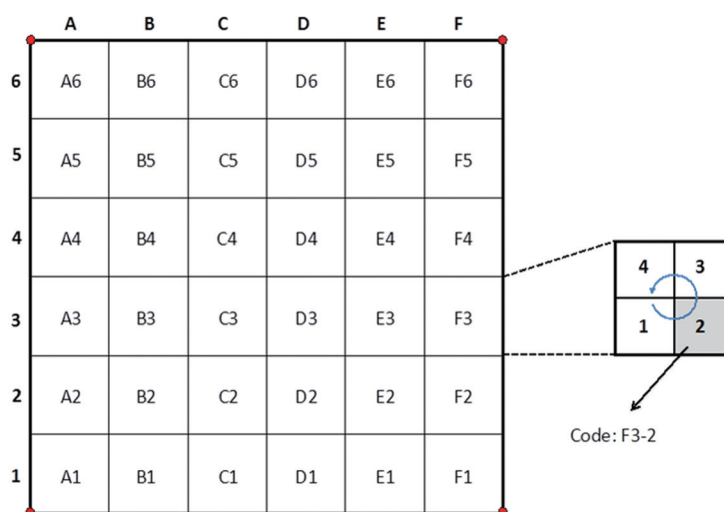
図 T13-3 プロットの区画例 たとえば図右の灰色部分の方形区のコードは F3-2 となる
