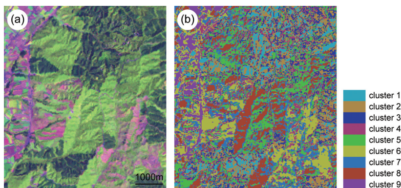
図 T09-1 ISODATA 法によるクラスターリング結果
