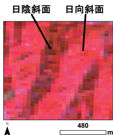
図 T07-2 日向斜面と日陰斜面の森林
