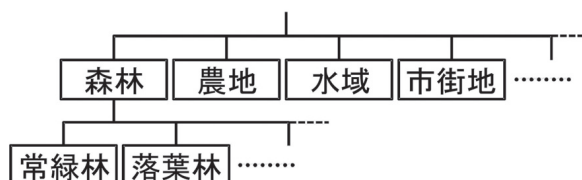
図 T07-1 クラスの階層構造
