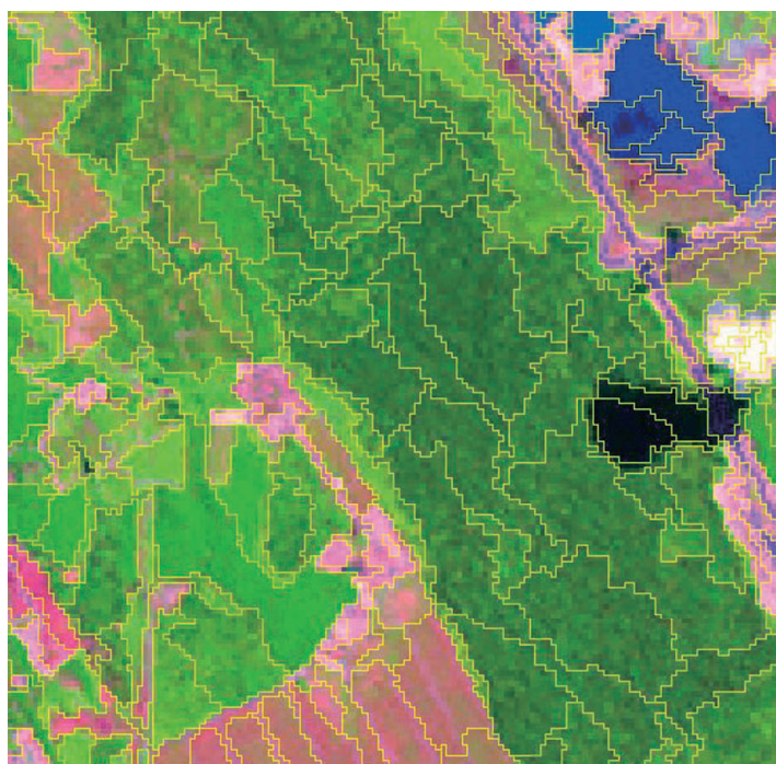
図 P08-2 Landsat 衛星画像のオブジェクトベース分類
