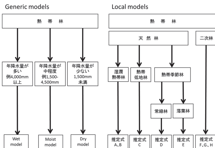
図 T14-2 アロメトリ式の推定フロー
