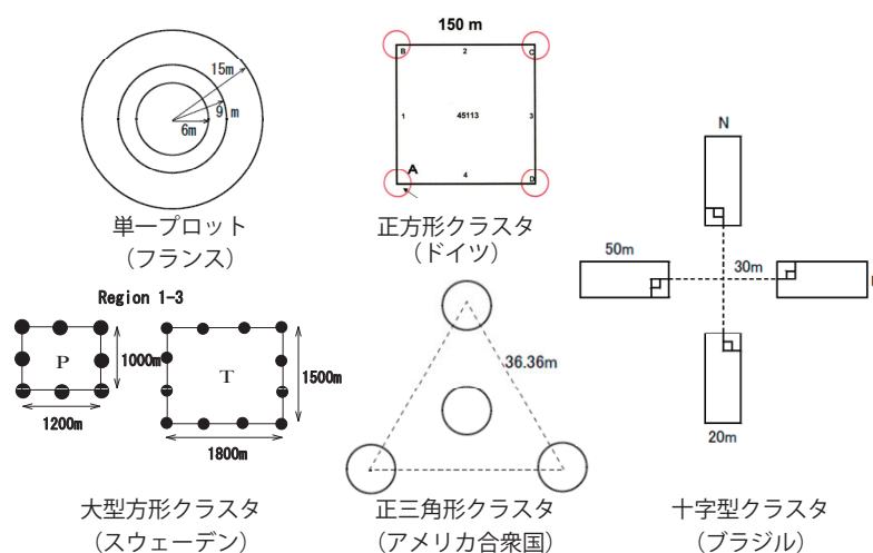
図 T01-2 国家森林資源調査におけるプロットの配置様式
