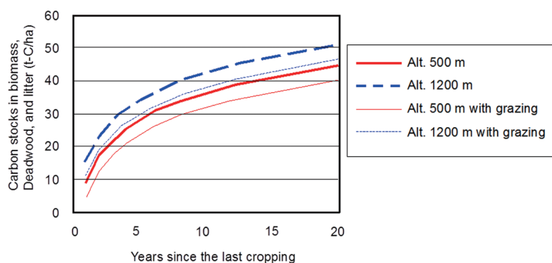
図 T18-1 休閑年数と炭素蓄積量の関係 (清野ら (2008) 3) を一部改変)
