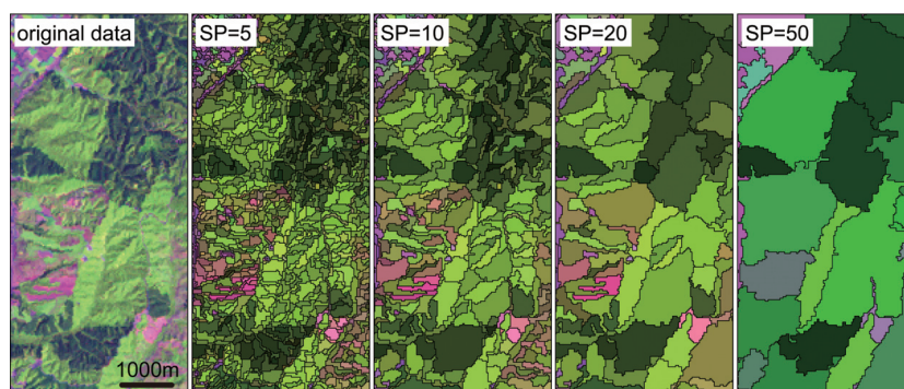
図 T09-2 オリジナルの Landsat ETM+ データと スケールパラメータ (SP) を変化させた時の領域分割結果
