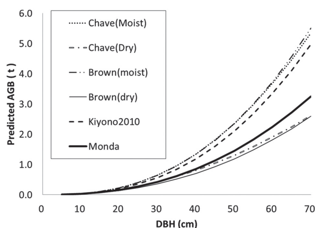
図 T14-1 推定式による地上部バイオマス (AGB: aboveground biomass) の推定値の違い 推定式とその出典は図 T14-2 を参照のこと。材密度 (WD) は 0.57 (Brown, 1997) を使用している
