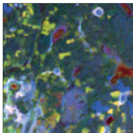
図 T11-2 2 時期の画像を併せた単一のマルチレイヤー画像 R：変化後画像バンド 3、G：変化後画像バンド 5、B：変化前画像バンド 5。森林→非森林への変化は黄色に、非森林→森林への変化は青く表示されている。
