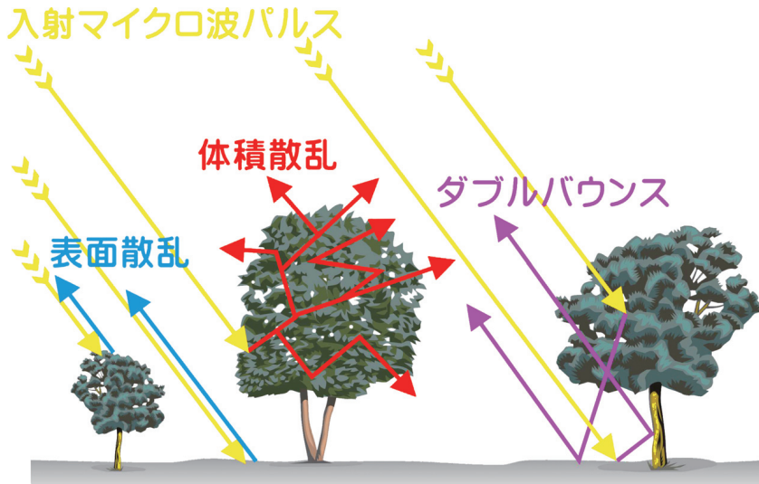
図 T05-1 森林における SAR 後方散乱の 3 成分
