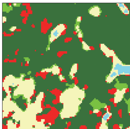
図 T11-1 2 時期それぞれの分類による変化抽出 緑：森林、黄：非森林、水色：水域、黄緑：非森林→森林、赤：森林→非森林、境界部分が変化として抽出されている。
