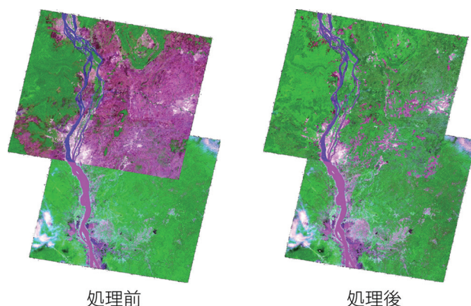
図 T06-3 季節変化の影響の除去の例 (Langner, 未発表) SPOT4 HRVIR 画像 (カンボジア)。上部の画像は既に乾季の最中だったために落葉樹林では落葉が進みピンクに見えるが、季節性を調整することにより落葉前の反射を復元でき、不自然な画像のつなぎ目も減少した。
