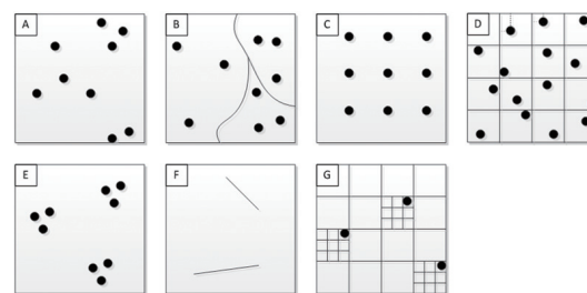
図 T08-1 抽出方法 A~G は表 T08-1 に対応
