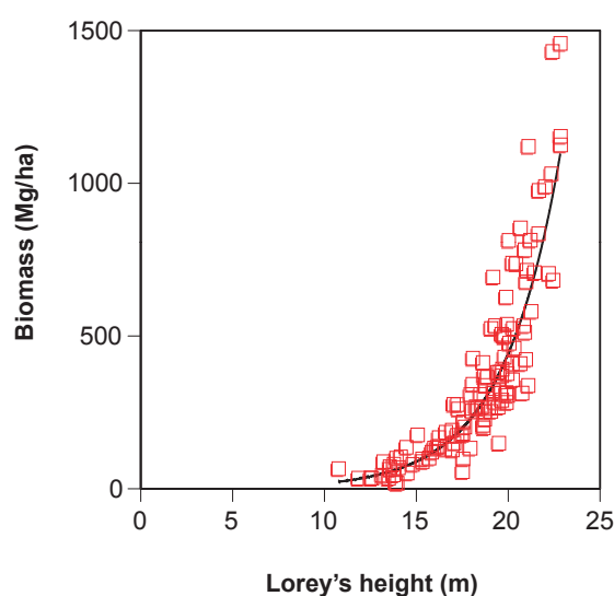
図 T16-1 胸高断面積により重み付けした平均樹高 (Lorey's height) とバイオマスの関係
