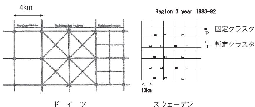
図 T01-1 国家森林資源調査におけるサンプリングのための格子の例
