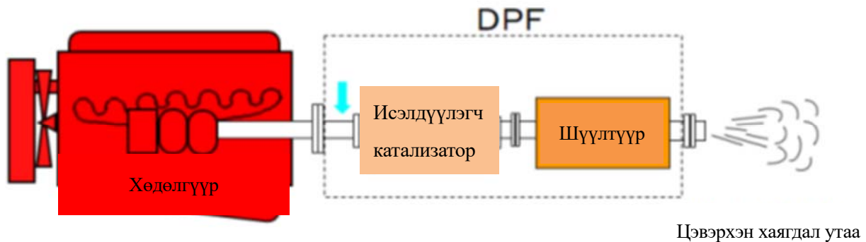
Зураг1 DPF-ын бүдүүвч
