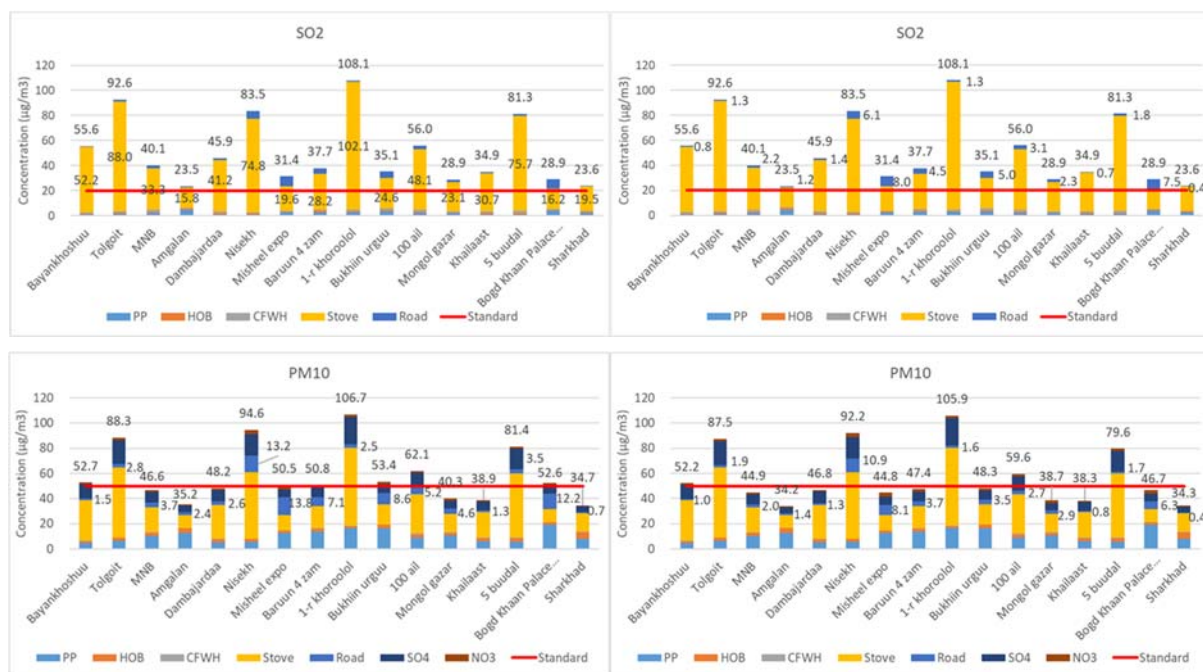
Зураг 4-8 Суурин харуулын жилийн дундаж агууламжийн бууралт (хэрэгжихээс өмнө ба дараах, эх үүсвэр тус бүрээр) /DPV, автобус/
