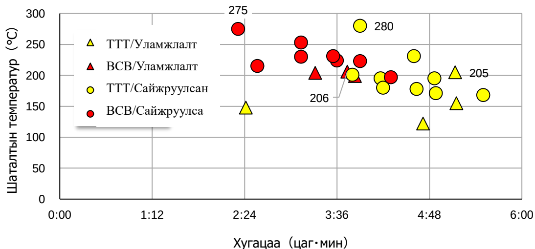
Зураг 3-7 Шаталтын хугацаа ба үүсэх температур
