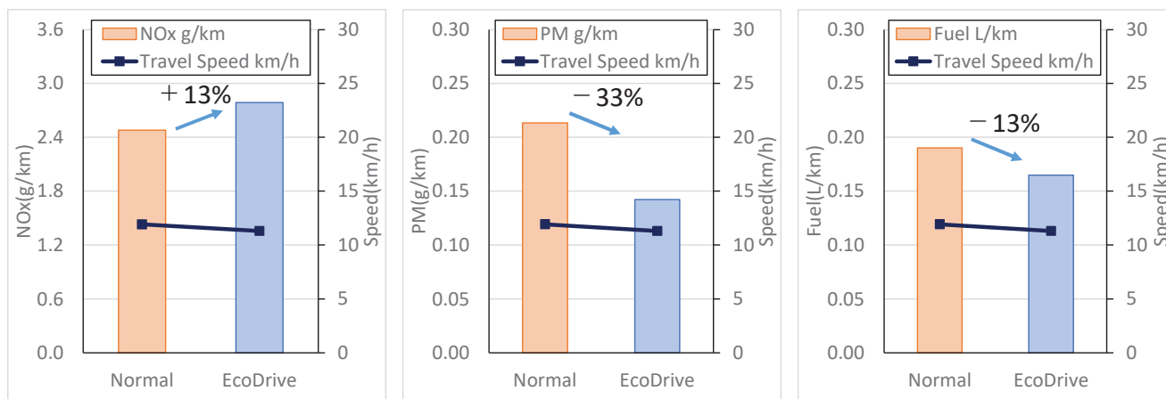
Зураг 1 (3): Эко жолоодлогоор агаар бохирдуулагчийг бууруулах үр нөлөө (Дизель ачааны машин)
