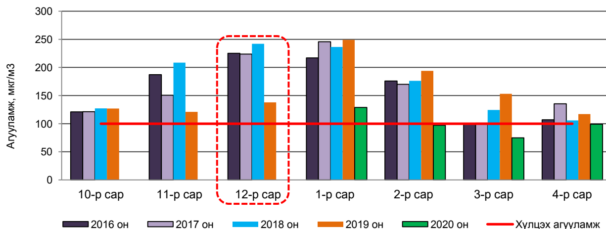
Зураг 16. Хүйтний улирлын PM10 тоосонцрын сарын дундаж агууламж, 2016-2020 он
