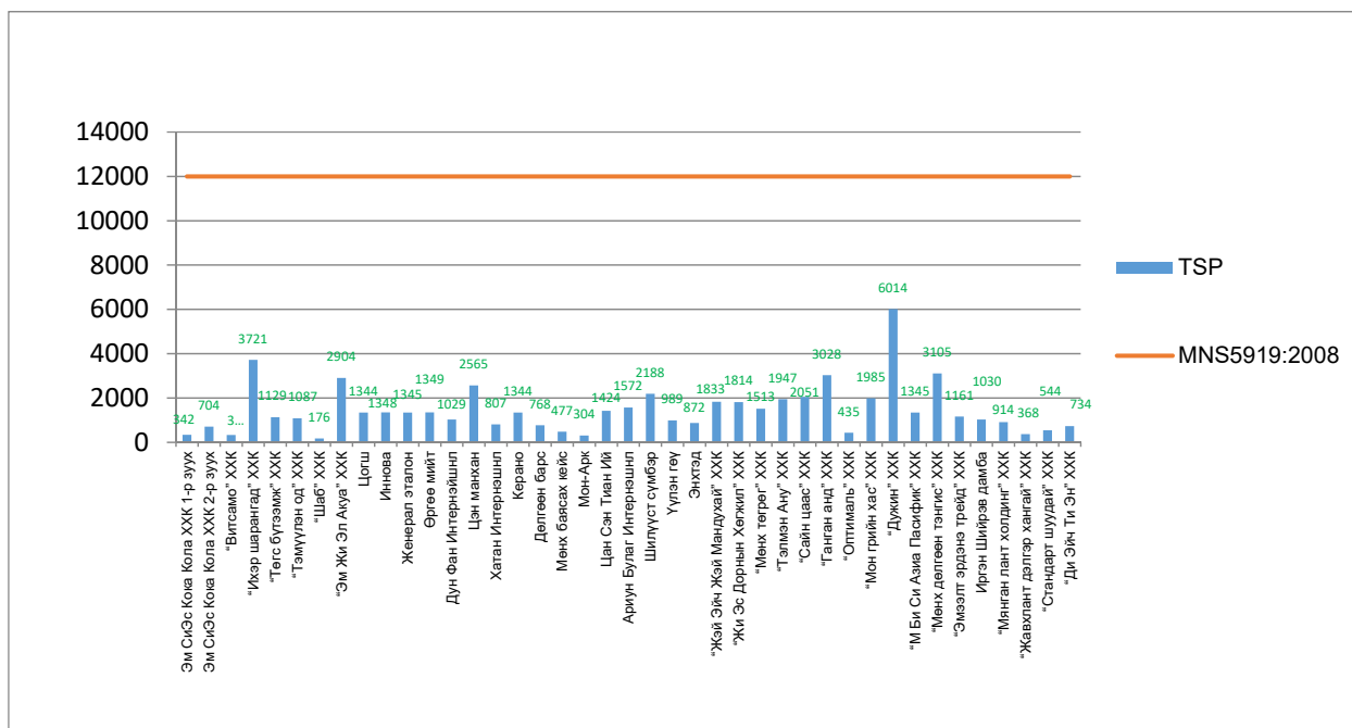
Зураг 29. Уурын зуухнуудын тоосонцор /TSP/-ын агууламжийн хэмжээ
