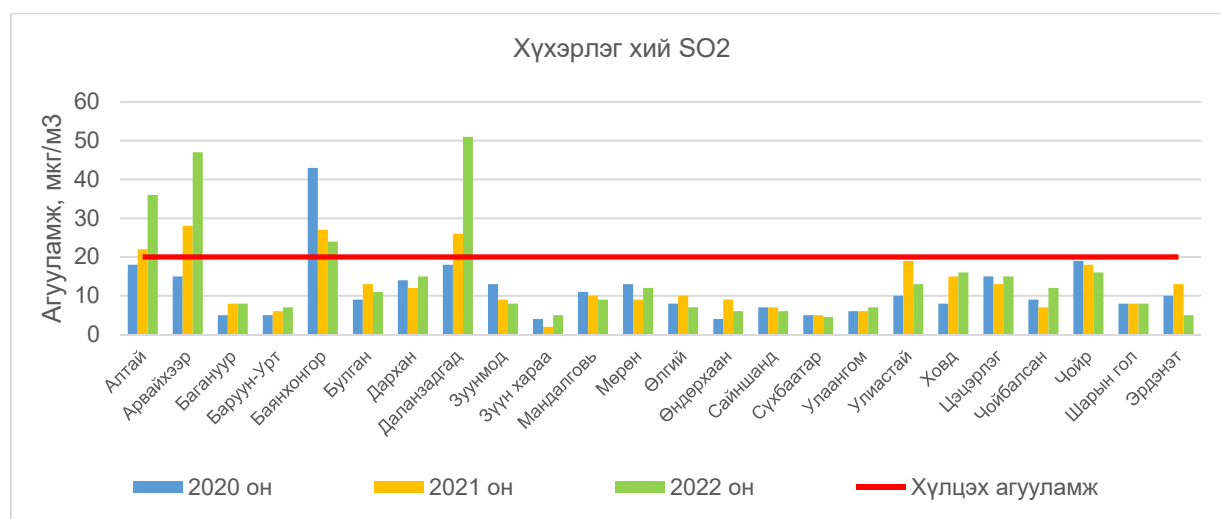
Зураг 21. Агаар дахь хүхэрлэг хийн жилийн дундаж агууламж
