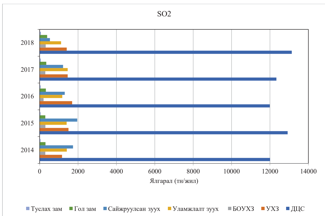
Зураг 9-2 SO 2 ялгарлын хэмжээний өөрчлөлт (эх үүсвэрээр)
