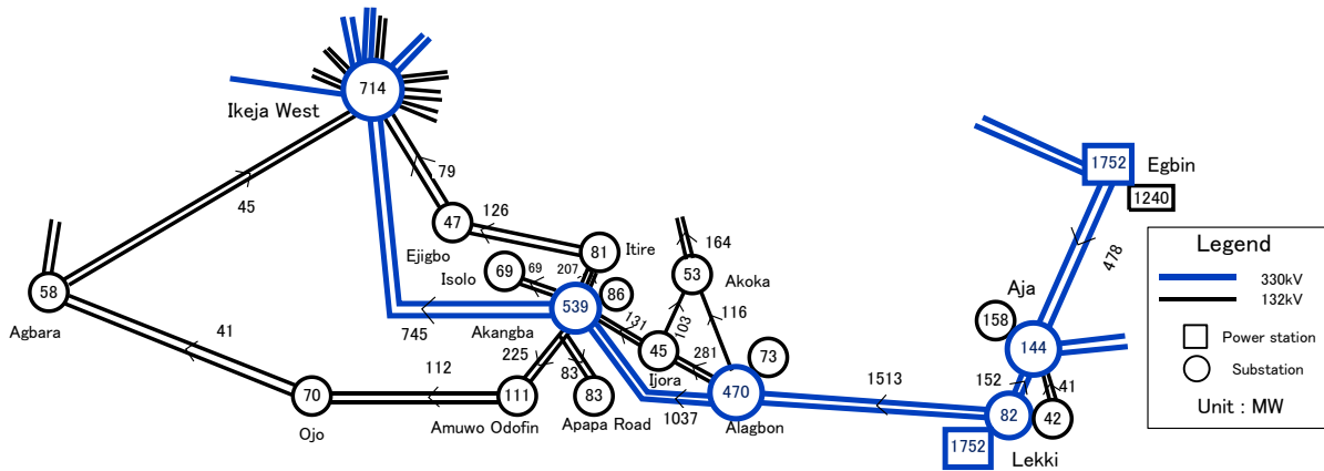
図 3-2-1 2 アパパロード変電所周辺系統の潮流状況（2025 年）
