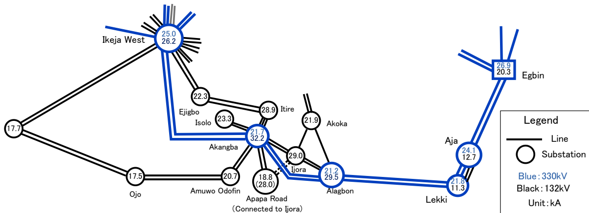
図 3-2-10 アパパロード変電所近傍の事故電流
