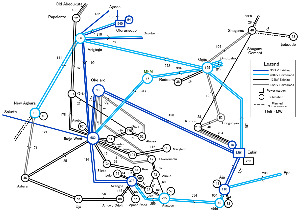
図 3-2-8 潮流解析結果 (2021 年)
