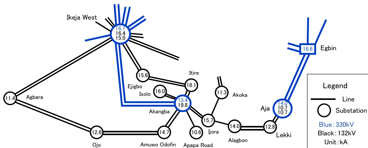
図 3-2-7 ラゴス系統の事故電流の現状
