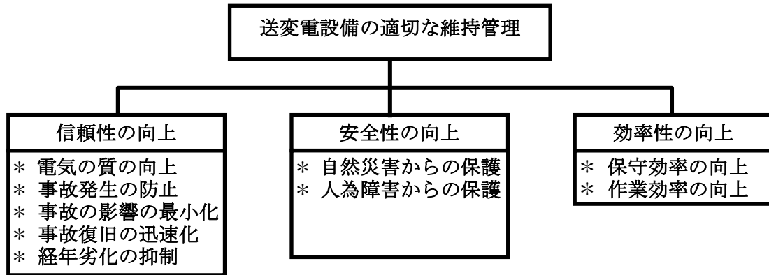
図 3-5-1 送変電設備の維持管理の基本的な考え方
