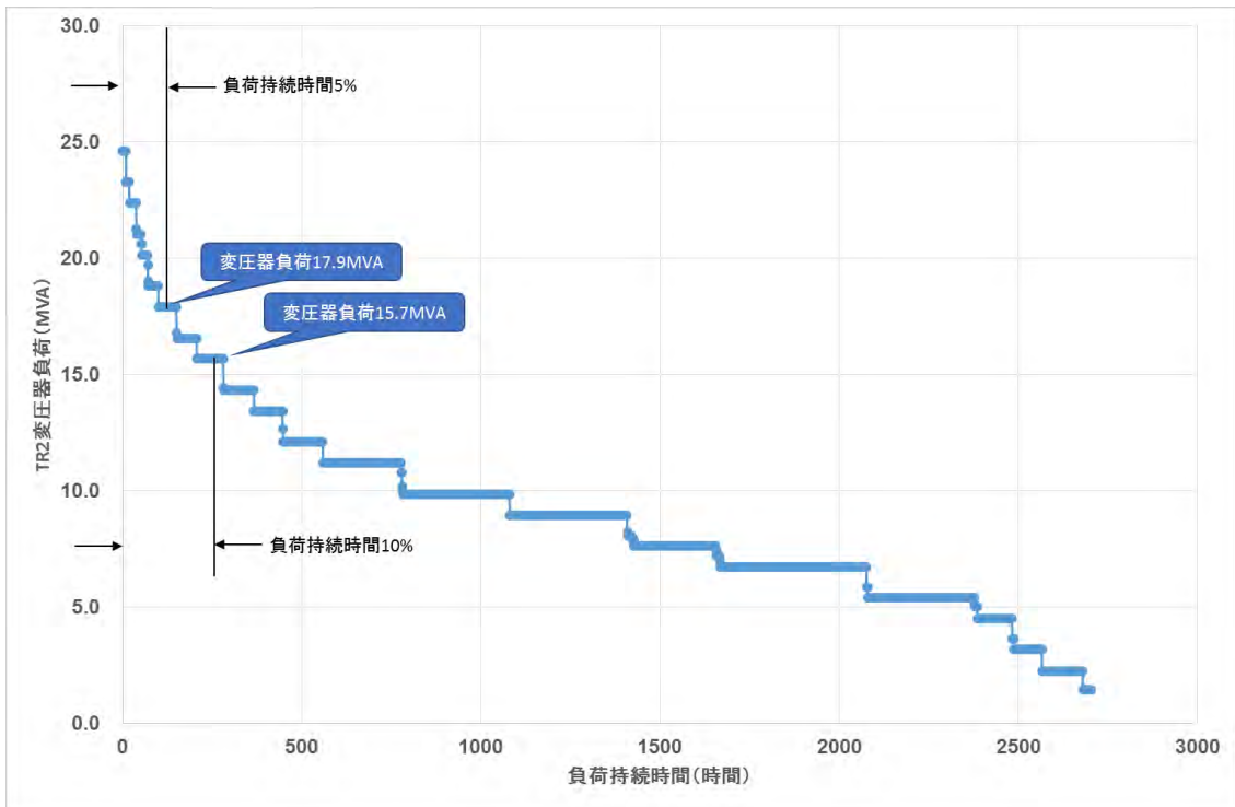
図 3-2-3 TR 2 変圧器負荷
