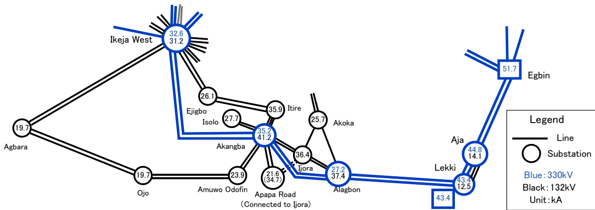
図 3-2-15 アパパロード変電所近傍の事故電流
