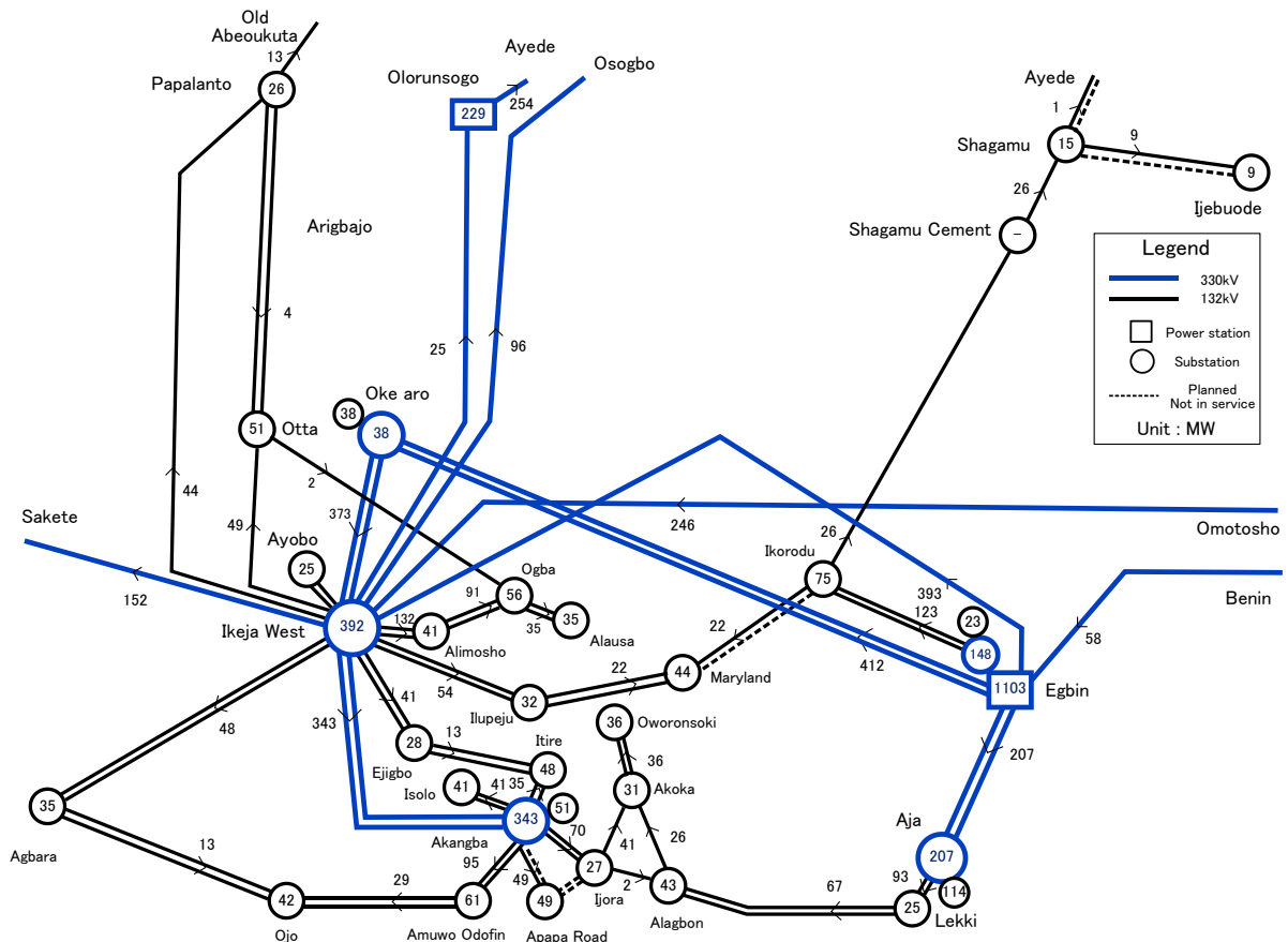
図 3-2-6 現状システムの潮流
