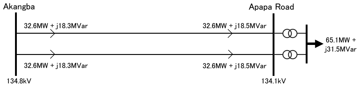
図 3-2-9 アカンバーアパパロード線の電圧および潮流状況
