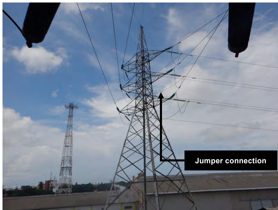
図 2-1-5 アカンバーアパパロード送電線のジャンパー接続部
