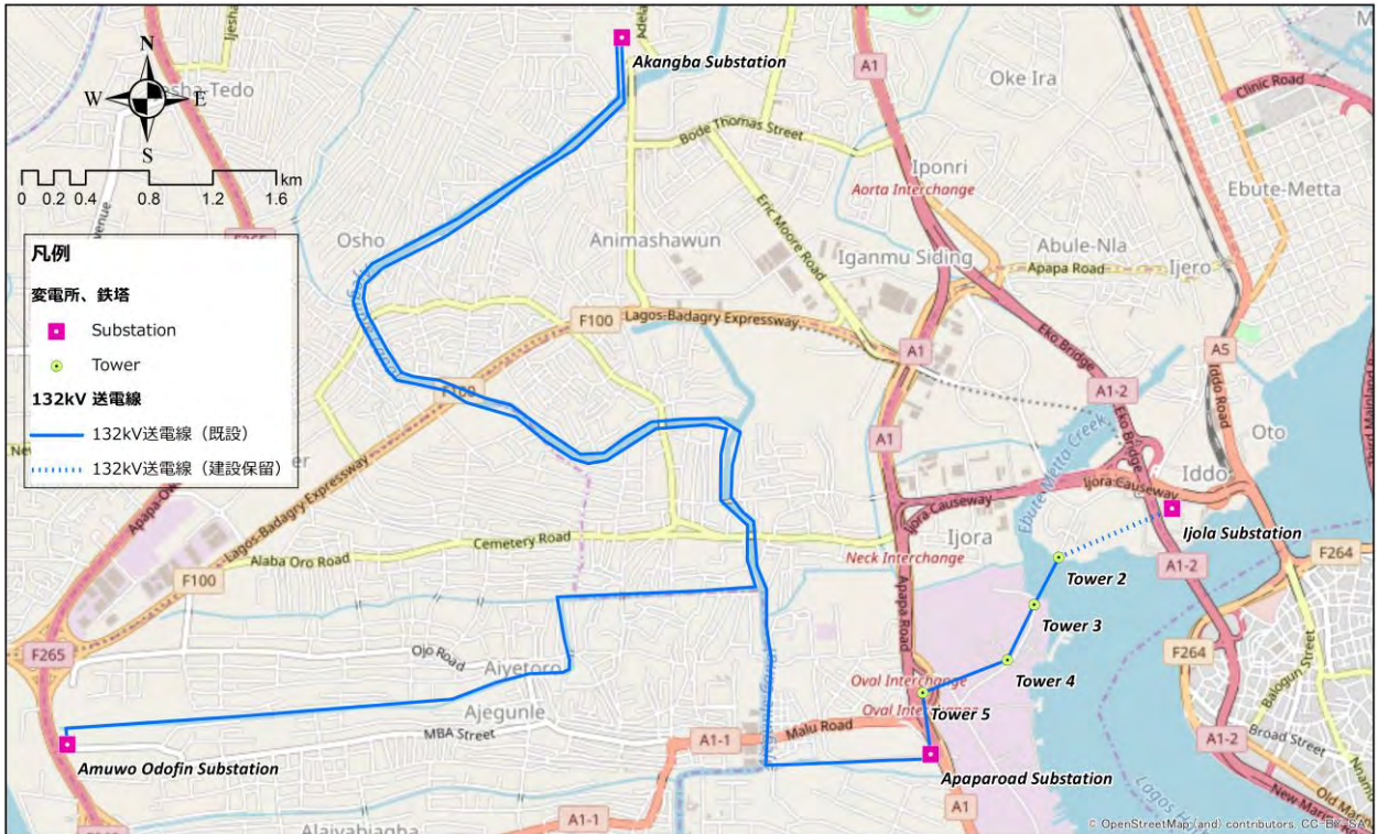
図 2-1-2 アパパロード変電所に接続する送電線
