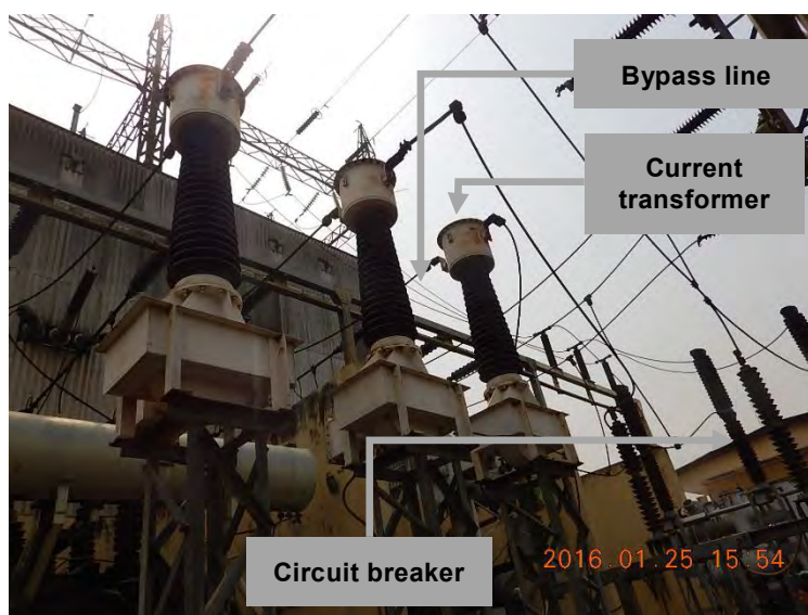
図 2-1-8 仮設開閉設備
