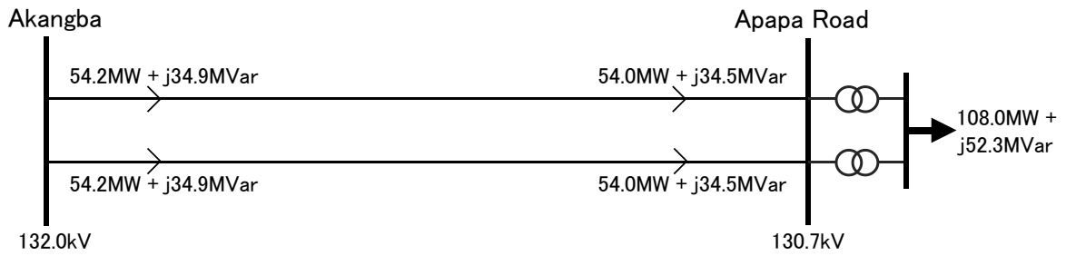
図 3-2-14 アカンバ変電所最終負荷時のアカンバーアパパロード線の電圧および潮流状況
