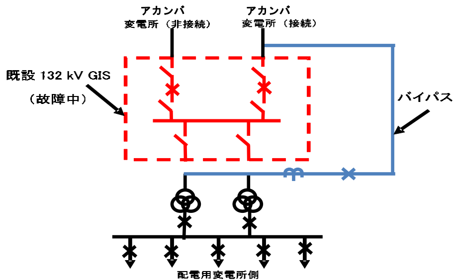
図 2-1-7 既設 132 kV GIS
