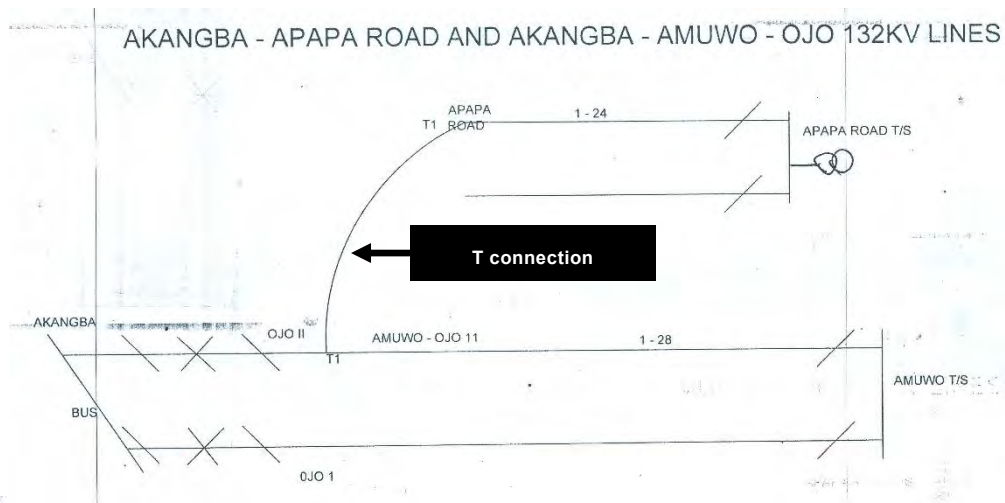
図 2-1-3 アカンバーアパパロード送電線の接続状況
