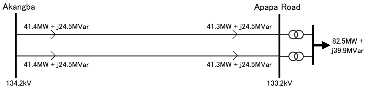
図 3-2-1 3 アカンバーアパパロード線の電圧および潮流状況
