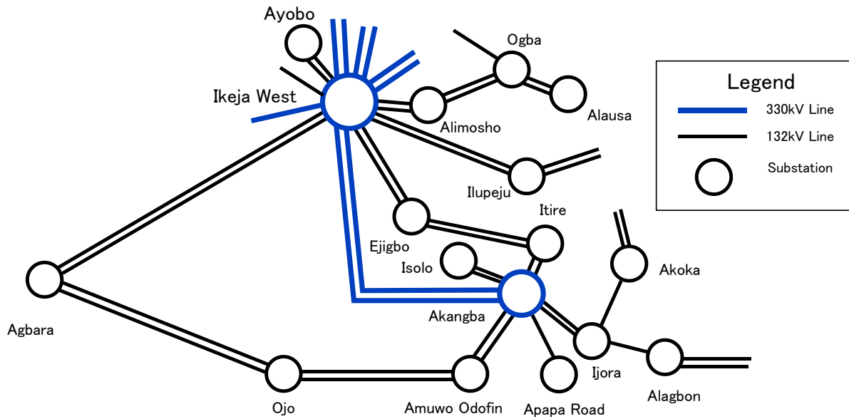
図 3-2-5 ラゴス州主要系統
