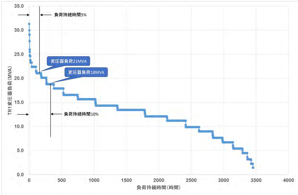
図 3-2-2 TR 1 変圧器負荷
