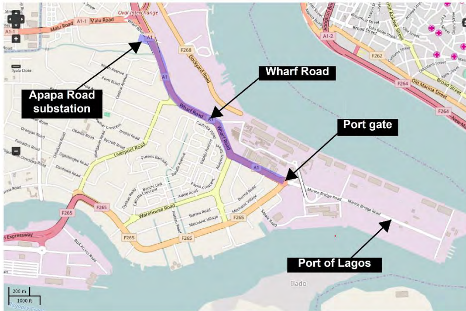
図 2-2-1 アパパロード変電所までの資機材輸送経路
