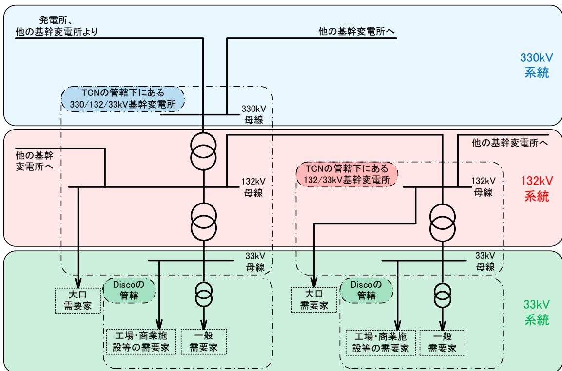
図 1-1-1 ナイジェリア送電系統の構成図
