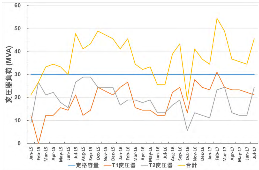
図 3-2-1 アパロード変電所の変圧器最大負荷実績 (2015年1月~2017年7月)
