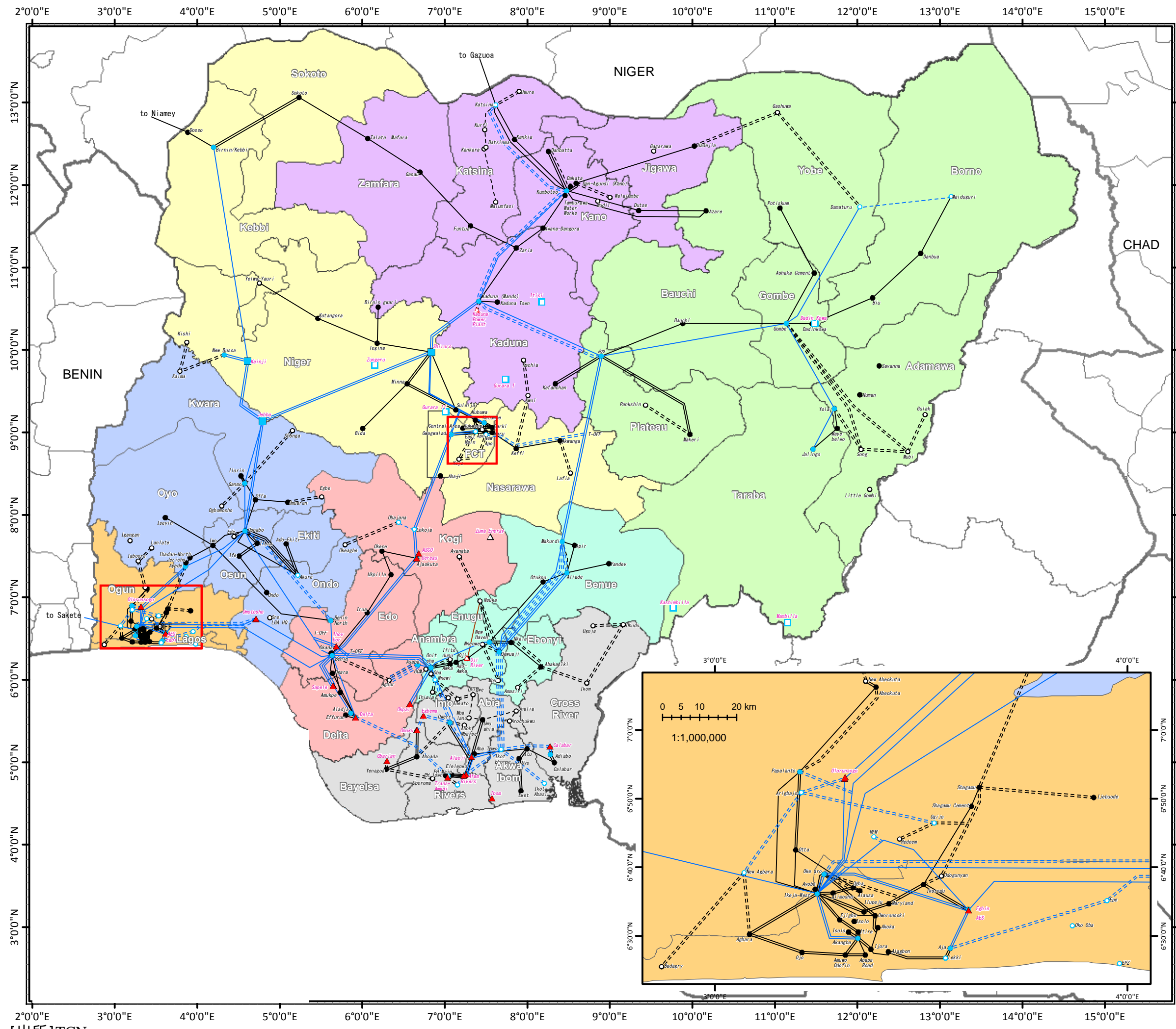
図 3-2-4 ナイジェリアの電力系統
