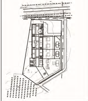
敷地全体図
