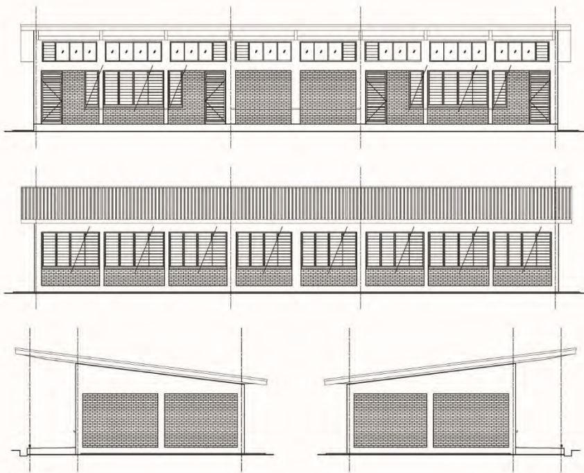
立面圖
