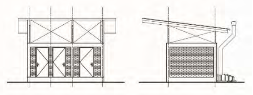
女子便所棟
